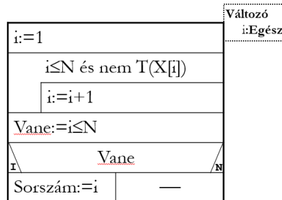
3. ábra. Lineáris keresés egy másik megvalósítása
