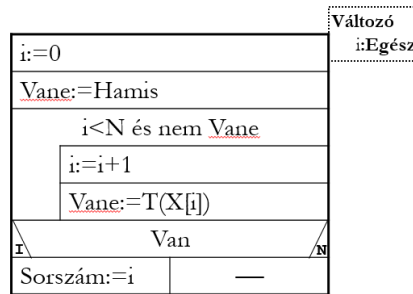
2. ábra. Lineáris keresés megoldása struktogrammal
