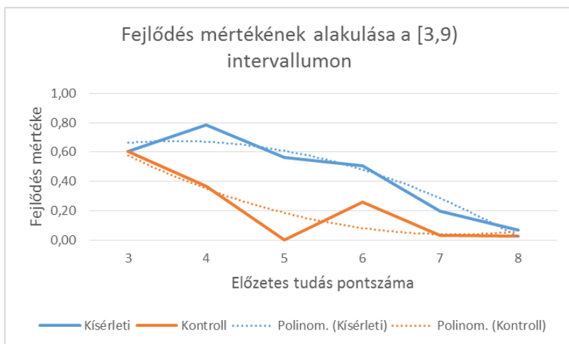
8. ábra. Fejlődés mértékének alakulása a [3,9) intervallumon.
