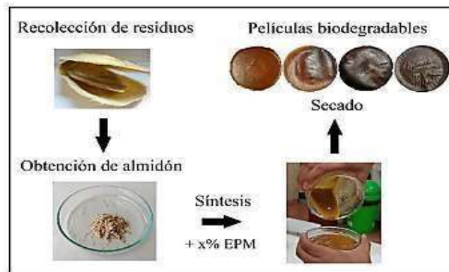
Figura 07. Proceso de elaboración del bioplástico de mango. Fuente: Naveda et, al 2020.
