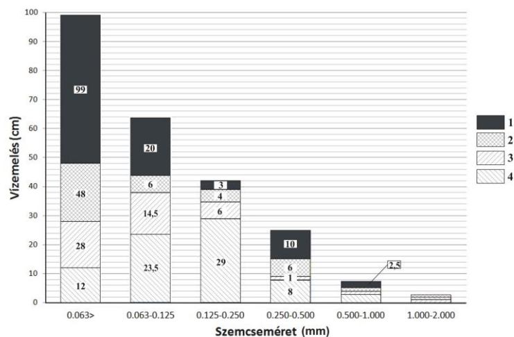
3. ábra: A vízemelő képesség alakulása különböző szemcseméretű üledékekben Jelmagyarázat: 1. Teljes vízemelés, 2. vízemelés 24 óra alatt, 3. vízemelés 5 óra alatt, 4. 1 óra időtartam alatti vízemelés.
