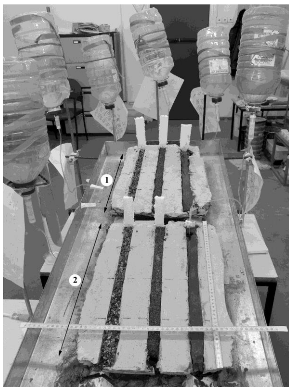
7. kép: A kísérleti hasadékok Picture 7: Experimentál grikes
