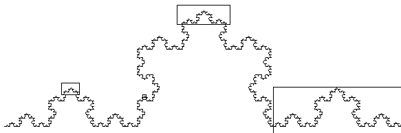
2. ábra. Önhasonlóság a tengerpartok vonalában 2
