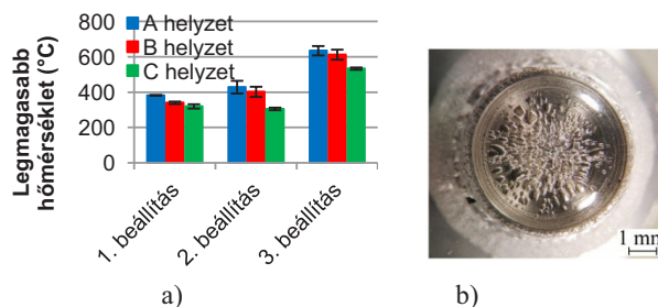
10. ábra. A csap pereménél mért legnagyobb hőmérsékletek a különböző helyzetek és beállítások esetén (a) és a csap homlokfelületénél megjelenő buborékok (b)
