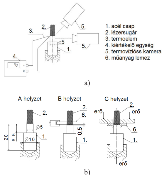
5. ábra. A hőmérsékletmérés vázlata termoelemmel és termovíziós kamerával (a), és helyzetek a PMMA acél hőmérsékletére gyakorolt hatásának vizsgálatához (b)
