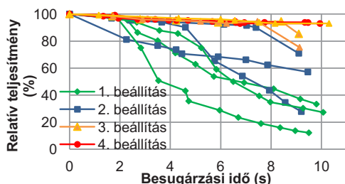
9. ábra. A lézerbeállítások hatása a PMMA áteresztésének változására
