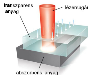
1. ábra. Lézeráteresztő hibrid kötés készítésének vázlatja [6]
