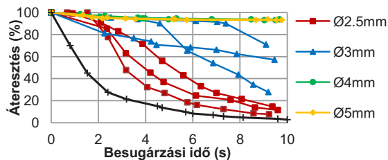
7. ábra. A PMMA áteresztésének változása különböző lézerező-átmérők esetén
