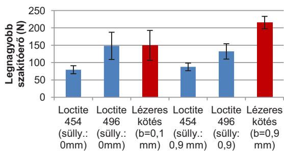
16. ábra. Ragasztott és LAMP eljárással készült kötések szakítóerejének összehasonlítása (b: benyomódási mélység)
