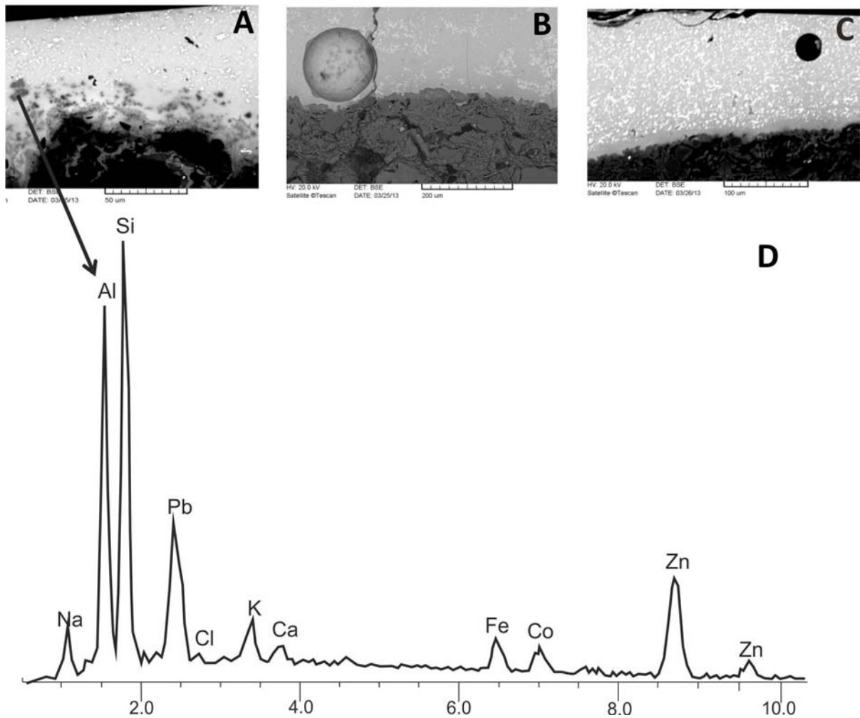
11. ábra: A Földtani Intézetről származó kerámiák mázrétegének zárványai. A nagy mennyiségben, elszórtan vagy rendezetlen csomókban megjelenő világos szemcsék ón-oxid zárványok. A) „idős” kerámia (1. csoport, MÁFI/10, visszaszórtelektron-kép), B) „középkorú” kerámia (2. csoport, MÁFI/2, visszaszórtelektron-kép), C) „fiatal” kerámia (3. csoport, MÁFI/15, visszaszórtelektron-kép). D) az „idős” kerámiát borító mázban az ón-oxid szemcsék mellett megjelenő cink-, vas- és kobalttartalmú szemcsék EDS spektruma
