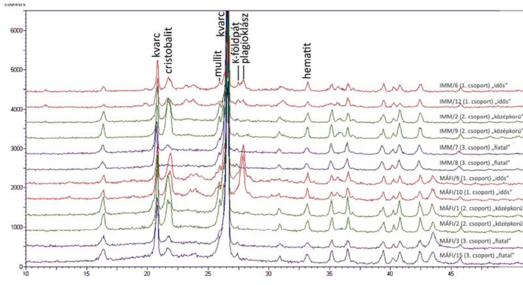
2. ábra: A kerámia-alaptestek röntgen-pordiffraktogramjai. Piros színnel az „idős” csoport, zöld színnel a „középkorú” csoport, kék színnel a „fiatal” csoport diffraktogramjai láthatók, amelyekben megfigyelhető a kvarc, cristobalit, mullit, K-földpát, plagioklász és hematit fázisok jelenléte és korszakonként eltérő mennyisége. IMM: az Iparművészeti Múzeum kerámiái, MÁFI: a Magyar Földtani és Geofizikai Intézet kerámiái
