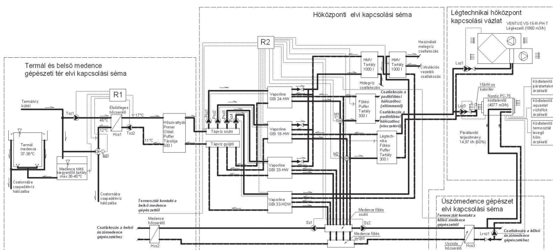
1. ábra. A nagykovácsi strandfürdő bővítése, gépezeti elvi kapcsolási rajz
