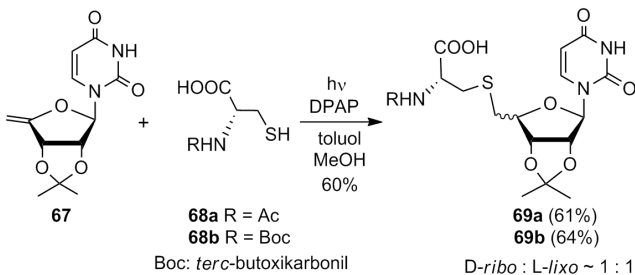
13. Ábra. Cisztein konjugálása uridinhoz fotokatalitikus tioladdícióval.
