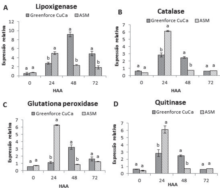
FIGURA 2 - Efeito dos tratamentos Greenforce CuCa e ASM em mudas de café. Expressão relativa dos genes que codificam para as enzimas lipoxigenase (A), catalase (B), glutaciona peroxidase (C), quitinase (D), nos tempos 0, 24, 48 e 72 horas, após aplicação dos tratamentos. Os genes GAPDH e o RPL7 foram usados como controle endógeno. Barras de erros representam o erro padrão da média de três repetições. As letras nas barras de erros representam a análise dos efeitos de cada produto aplicados ao longo do tempo, conforme Tukey, a 5% de probabilidade.
