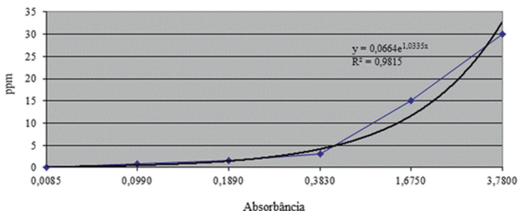
FIGURA 1 - Curva de leitura de absorbância para inferir a concentração (ppm de corante) das amostras de calda. Monte Santo de Minas/MG. Ano agrícola 2010/2011.
