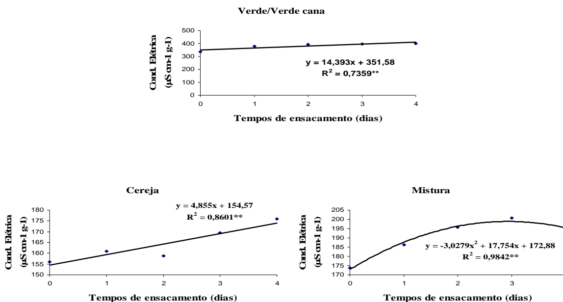
Figura 1 – Teores de condutividade elétrica ( \mu\text{S cm}^{-1} \text{g}^{-1} ), em cafés ( Coffea arabica L.) dos estádios de maturação verde/verde cana e cereja e fração mistura submetidos a diferentes tempos de ensacamento antes da secagem.
