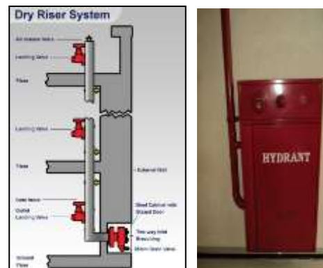
Gambar 6. Sistem Pipa Tegak di Gedung Rektorat Undana
