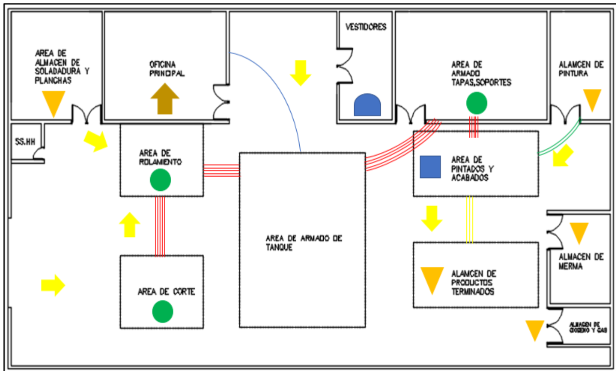
Figura 9: Layout Propuesto para Industrias Metálicas El Sol. Elaboración Propia.
