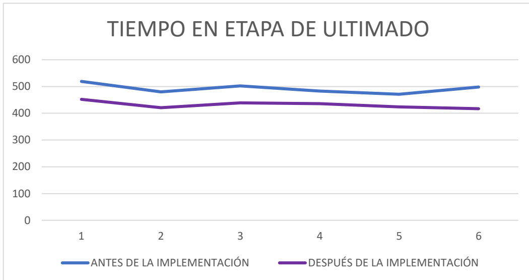
Figura 15: Comparación de tiempo en etapa de ultimado de la Empresa Metálicas El Sol. Elaboración Propia.
