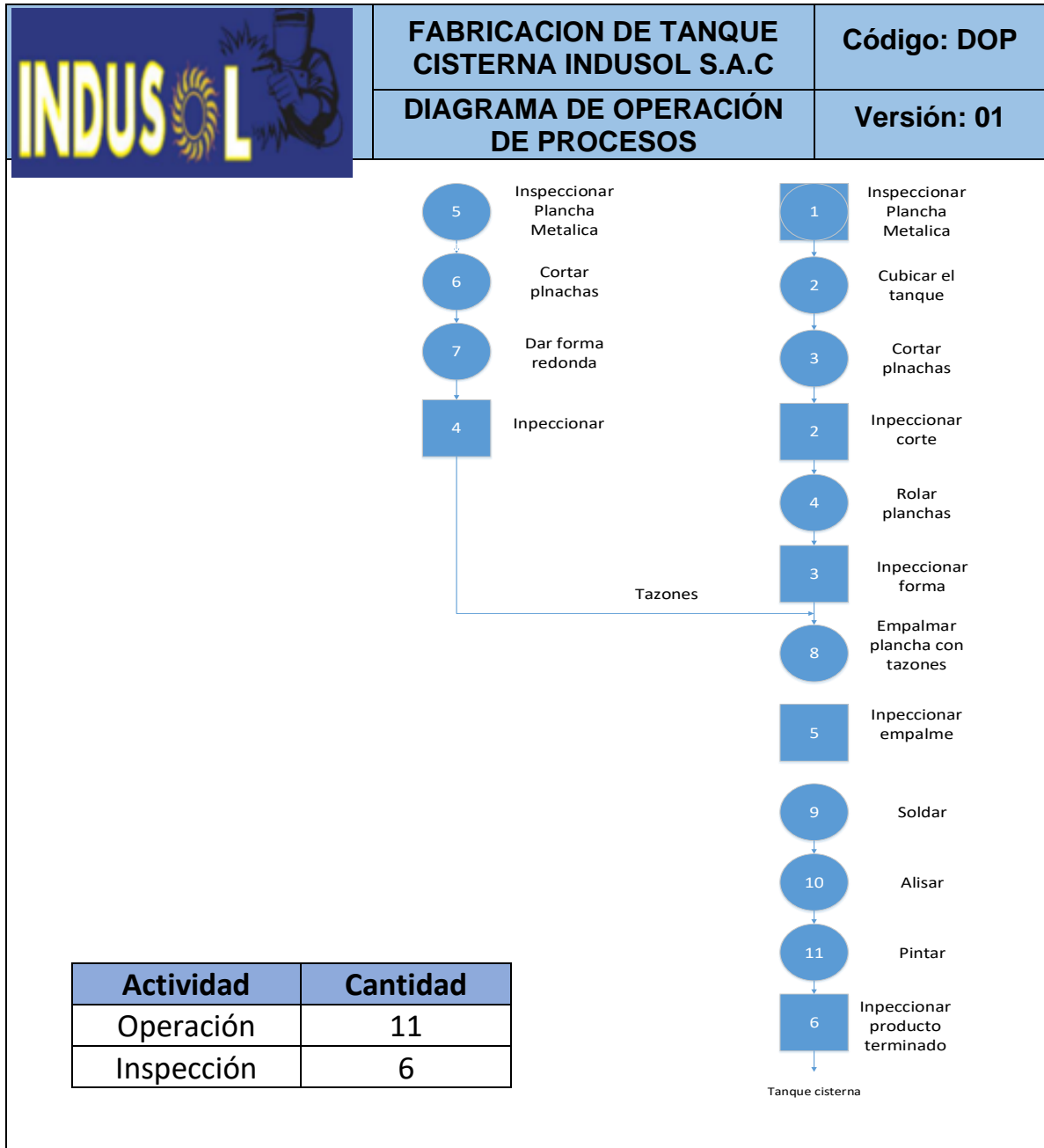
Figura 6: Diagrama de operaciones del proceso en Industrias Metálica El Sol. Elaboración Propia
