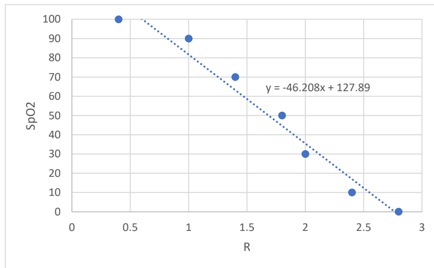
Figura 13. Curva de calibración del Oxímetro de Pulso Fuente: Elaboración Propia
