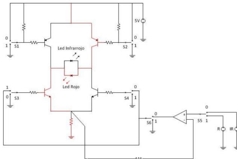
Figura 1. Esquema circuitos para el manejo de corrientes de LEDs
