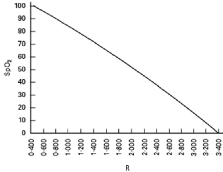
Figura 12. Valores de saturación de oxígeno vs absorbancia Fuente: Aguirre Luis, 2007
