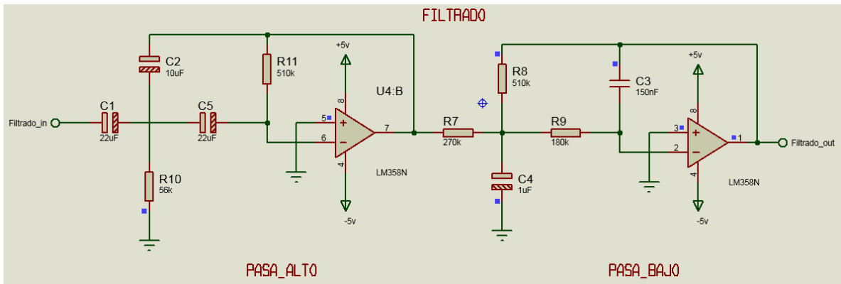
Figura 21. Filtro pasabanda Fuente: Elaboración Propia
