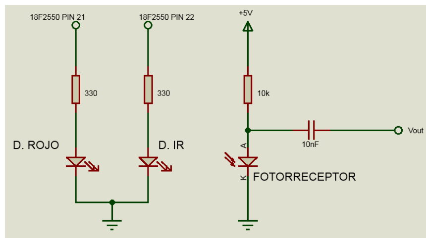
Figura 34. Captación de Señal Fuente: Elaboración Propia
