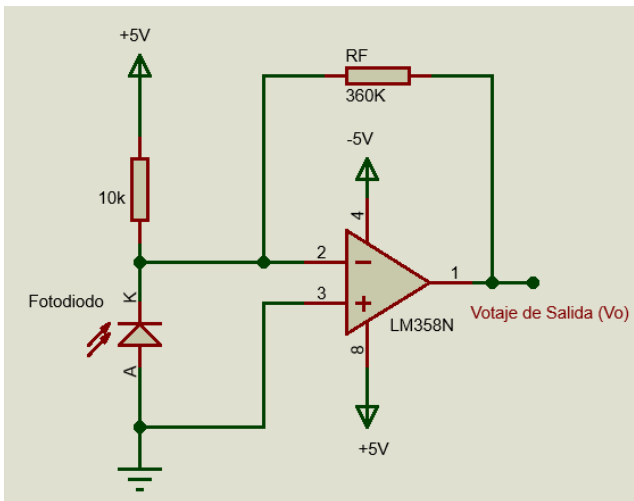
Figura 35. Circuito de transimpedancia y Amplificación Fuente: Elaboración Propia
