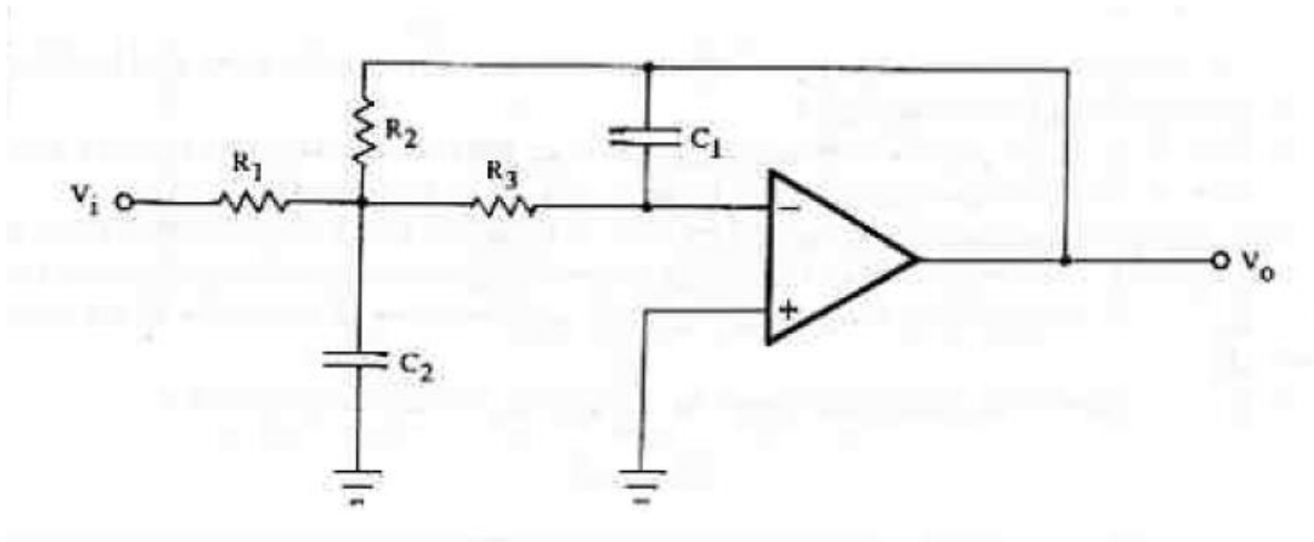
Figura 11. Filtro pasa bajo
