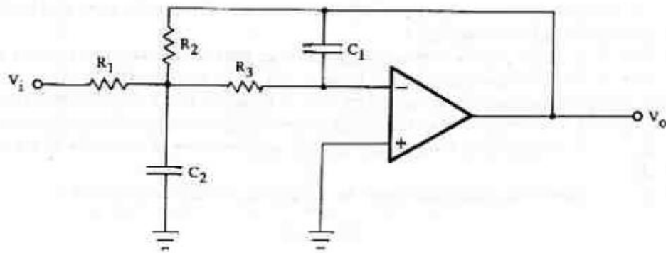
Figura 7. Filtro pasa bajo Fuente: Antonio Pertence Junior, Amplificadores Operacionales y filtros activos
