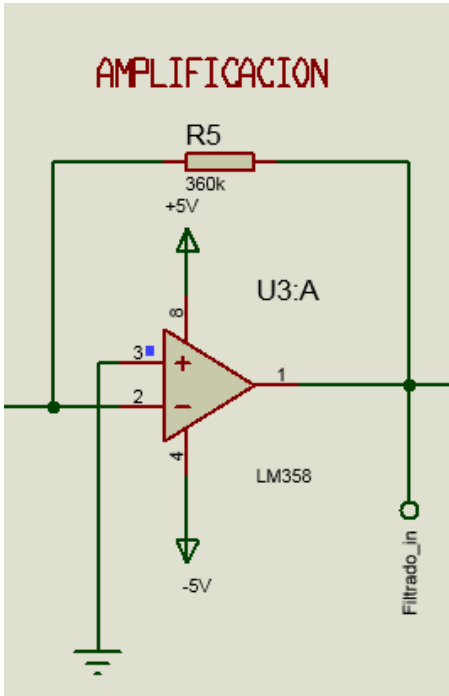
Figura 20. Diagrama de amplificación Fuente: Elaboración Propia
