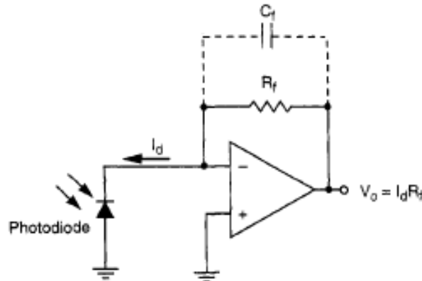
Figura 2. Circuito amplificador de transimpedancia Fuente: Antonio Pertence Junior, Amplificadores Operacionales y filtros activos
