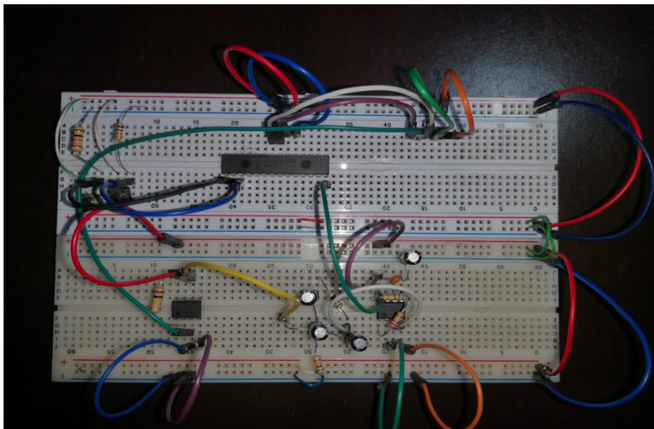
Figura 41. Oxímetro de Pulso, circuito en Protoboard Fuente: Elaboración Propia
