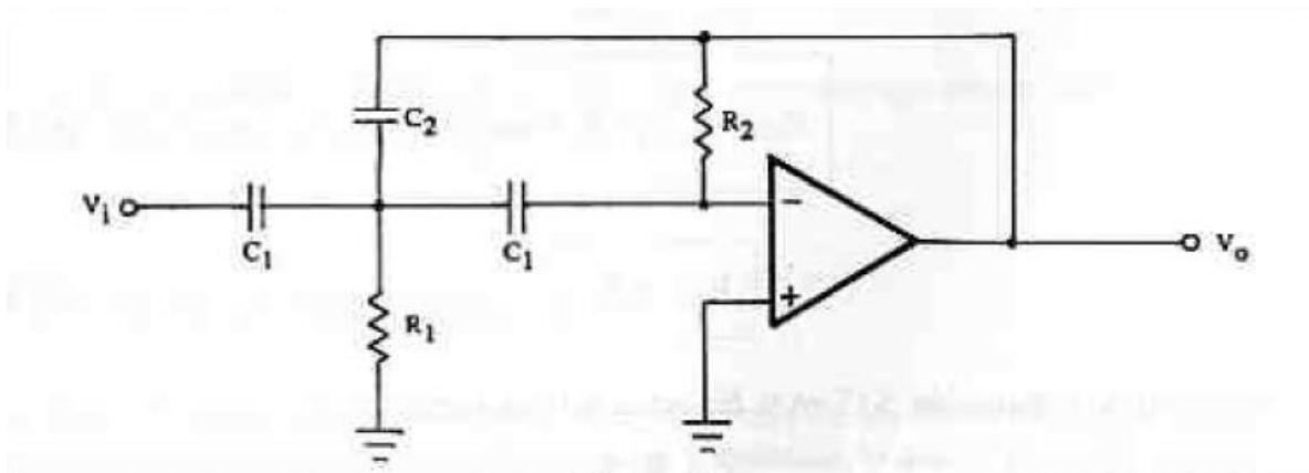
Figura 10. Filtro pasa alto Fuente: Antonio Pertence Junior, Amplificadores Operacionales y Filtros Activos
