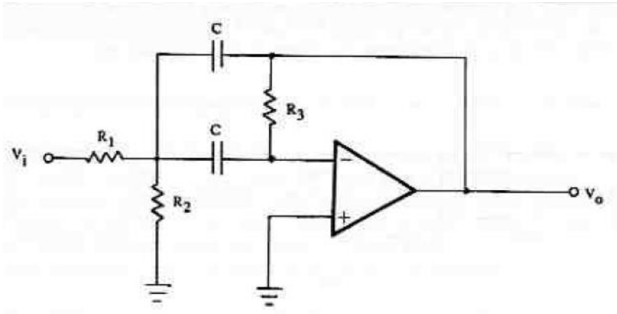
Figura 4. Circuito MFB Filtro pasabanda Fuente: Antonio Pertence Junior, Amplificadores Operacionales y filtros activos
