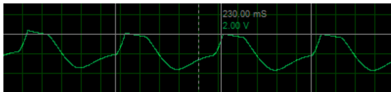
Figura 22. Señal de salida después del filtrado
