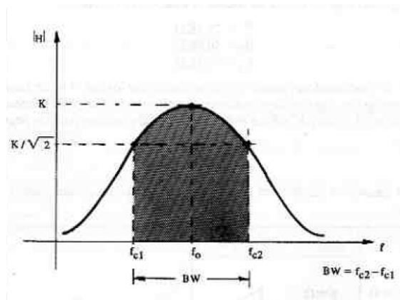
Figura 3. Filtro pasabanda Fuente: Antonio Pertence Junior, Amplificadores Operacionales y filtros activos
