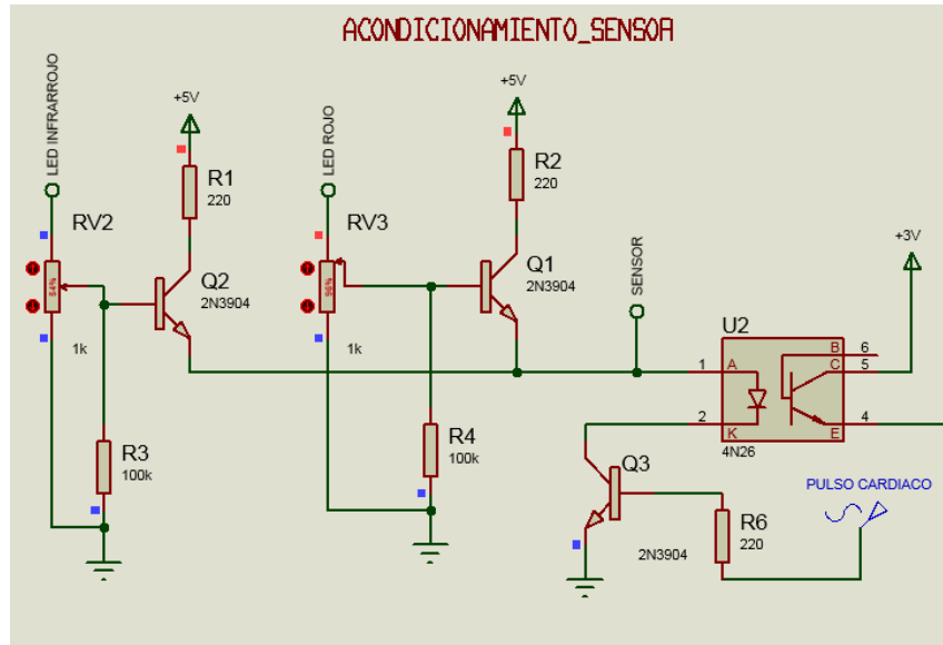
Figura 18. Captación de Señal o Acondicionamiento del Sensor Fuente: Elaboración Propia
