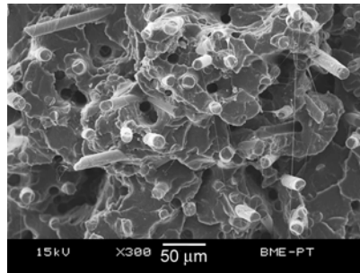
8. ábra. 25,8 m% rövid bazaltszállal erősített fröccsöntött próbatestet törtet-felülete
