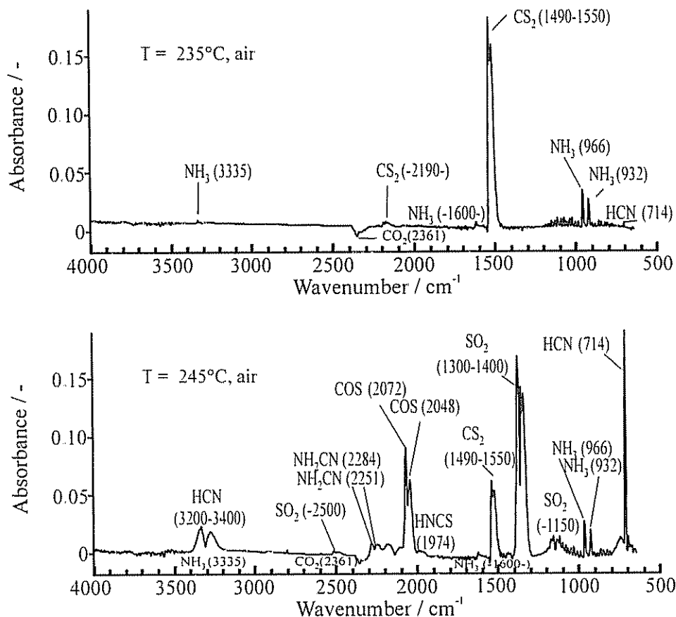
3. Ábra. ZnS filmek porlasztásos pirolízises előállítására ajánlott, 49 (Zn- és S-tartalmú) egyforrású \text{Zn}_2(\text{tiokarbamid})_2\text{Cl}_2 prekursor vegyület termikus bomlása során keletkező gőzök és gázok FTIR spectrumai egy on-line kapcsolt TG-FTIR-gázcellás mérőrendszerrel in situ mérve. A 235°C-on intenzíven keletkező széndiszulfid ( \text{CS}_2 ) (felső spektrum) az áramló levegőben meggyullad és 245°C-on már az égéstermékai, úgymint kén-dioxid ( \text{SO}_2 ) és karbonil-szulfid ( \text{COS} ) jelennek meg, ill. hidrogén-cianid gáz, \text{HCN} intenzív fejlődése is tapasztalható (also spektrum), (fűtési sebesség 10^\circ\text{C min}^{-1} , kezdeti mintatömeg 24,10 mg, az interferogramok kumulálási ideje kb. 30 s) 41
