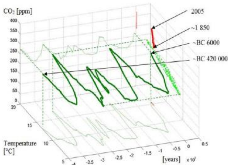
3. ábra Átlagos légköri CO 2 koncentráció és átlagos Földi középhőmérséklet complex idősorai (forrás: Tanczos, Torok, 2007)
