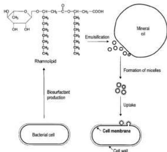
Figura 3. Involment of biosurfactants in the up-take of hydrocarbons (Fritsche și Hofrichter, 2008)
