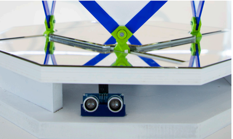
Fig. 47. Ultrasonic sensor.
