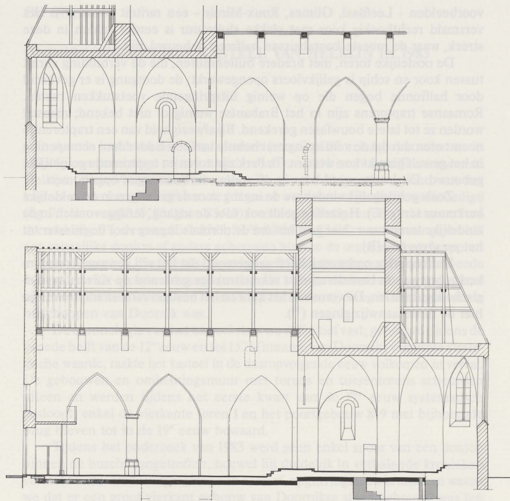
Fig. 76. Architecturale doorsneden, genomen op de lengteas (boven: naar het Z., onder: zicht naar het N.).
