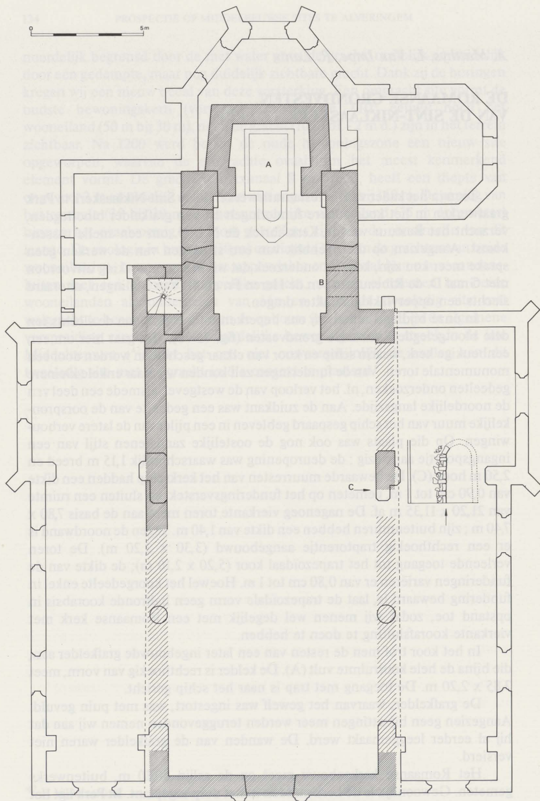
Fig. 75. Grondplan van de Romaanse kerk te Perk.
