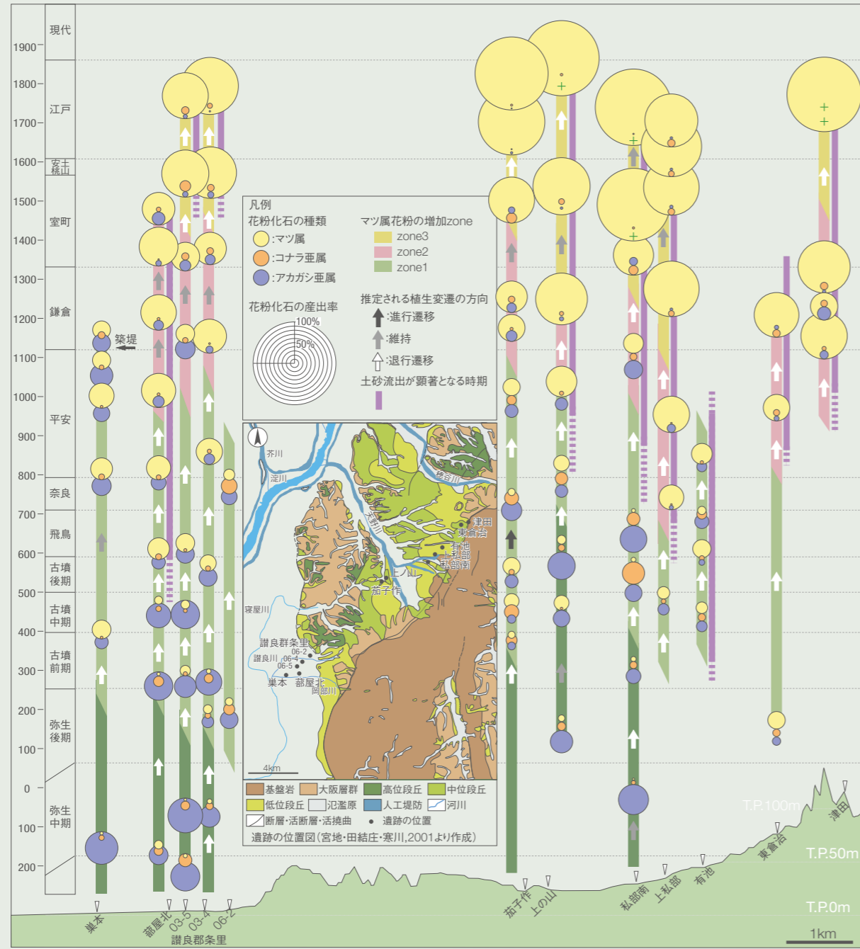
図2 生駒山西麓北部と枚方丘陵における古墳時代以降の主要花粉化石の変遷 (辻本 (2010) | 第27回日本文化財科学大会大会ポスター発表資料を引用・改変)
