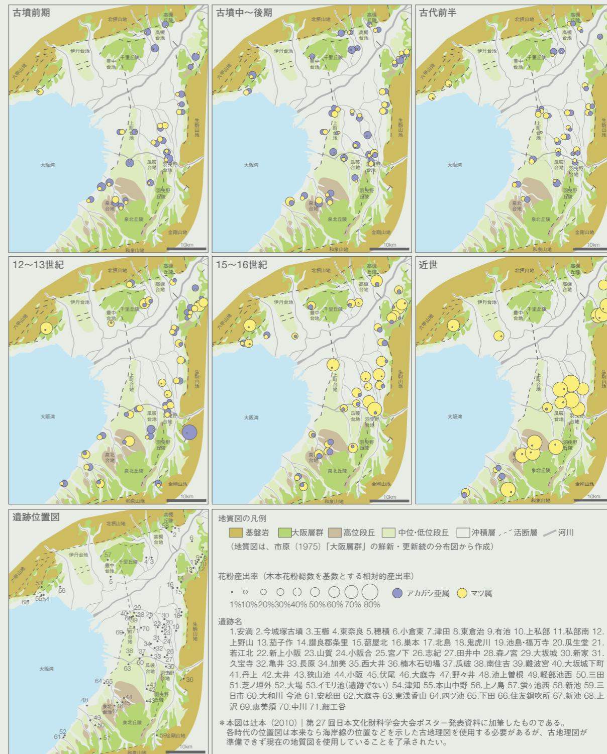
図1 大阪湾岸域の考古遺跡における古墳時代以降のアカガシ亜属・マツ属花粉の産出率の空間分布
