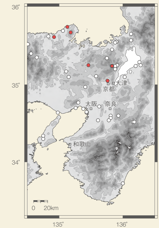
図1 近畿地方の湿原・湖沼堆積物による花粉分析地点(丸印)。このうち赤い丸印は、本文中で紹介した分析地点。高原(1998)がまとめた地点データの一部加筆し、ETOPO1 Global Relief Model (Amante and Eakins, 2009)を利用して作成
