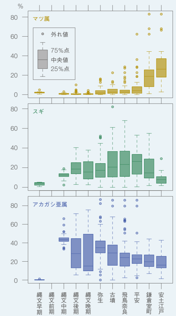
図2 滋賀県APPALeデータベースの花粉分析データに基づく主要花粉分類群の出現率変化(高木花粉総数を基数として算出)。林(2018)に基づいて作成
