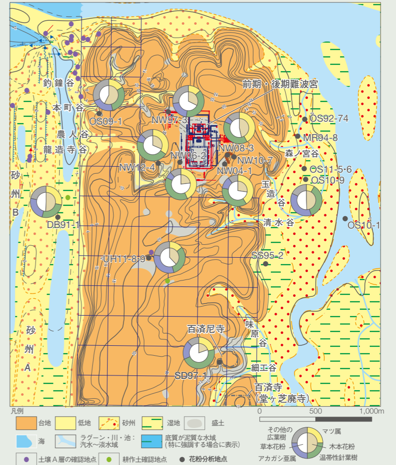
図3 上町台地北部における7世紀頃の花粉組成 (ベースマップは趙(2014)による「古代の古地理図」を引用・改変)
