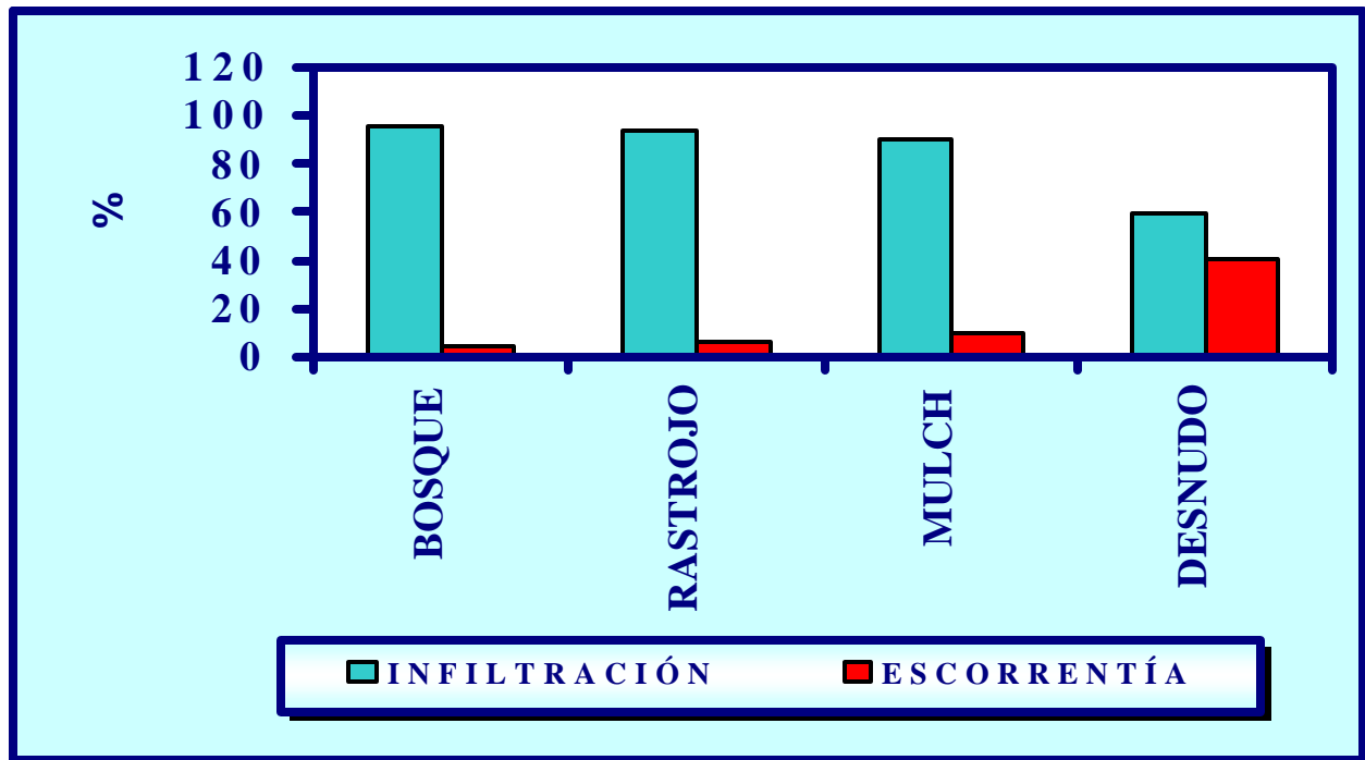
FIGURA 11.6. Efecto de la cobertura de un Ultisol de Florencia (Caquetá) sobre su relación infiltración – escorrentía, con respecto a la precipitación promedio anual (2900 mm); promedios de 12 años de observaciones. (Con base en resultados de Escobar et al, 1993).
