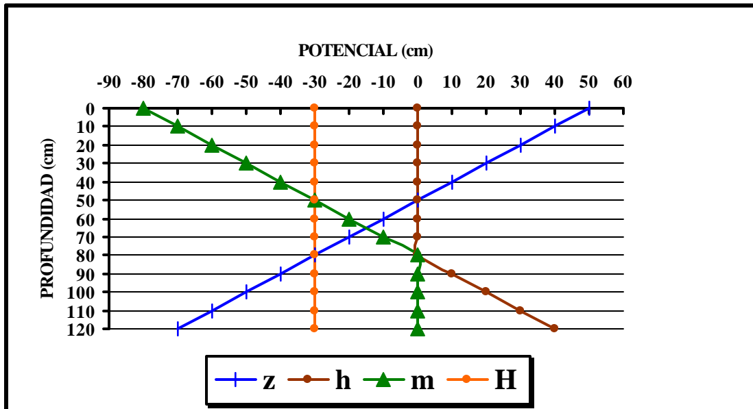
FIGURA 9.4. Comportamiento de las cabezas de potencial en un suelo hipotético cuya agua está en equilibrio. (Con base en los datos de la Tabla 9.1).
