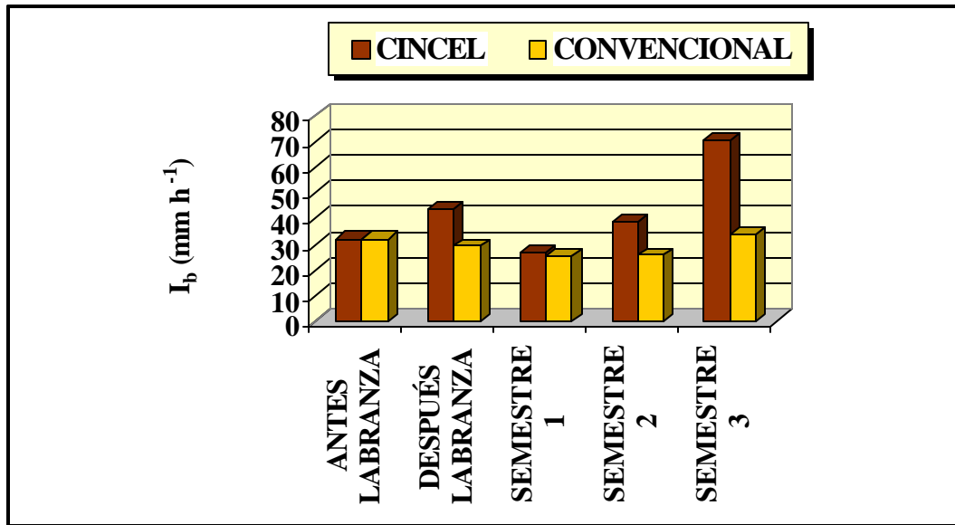
FIGURA 11.5. Efecto de diferentes sistemas de labranza, en el tiempo, sobre la infiltración básica de un suelo arenoso franco compactado de El Espinal (Tolima). (Con base en resultados de Castro y Amézquita, 1991).
