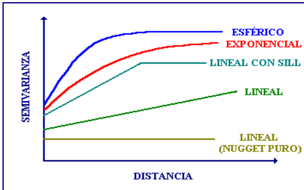
FIGURA 23.3. Modelos de semivariogramas comunes en propiedades de suelos.
