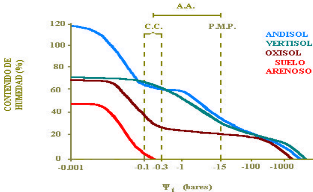
FIGURA 9.2. Efecto del tipo de arcilla del suelo, sobre su capacidad de retención de humedad (Contenido gravimétrico de humedad; A.A.: Agua aprovechable; C.C.: Capacidad de campo; P.M.P.: Punto de marchitez permanente). (Adaptada y complementada de varios autores, citados por Sánchez, 1981).
