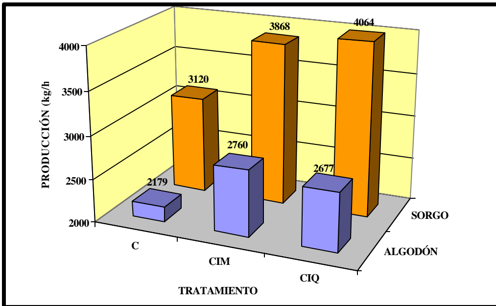
FIGURA 11.4. Efecto de diferentes sistemas de labranza de un Arenic Haplustalfs de EL Espinal (Tolima), sobre la producción promedio de dos semestres de algodón y sorgo sembrados en él. Para significado de los tratamientos, ver Figura 11.2. (Con base en resultados de Castro y Amézquita, 1991).
