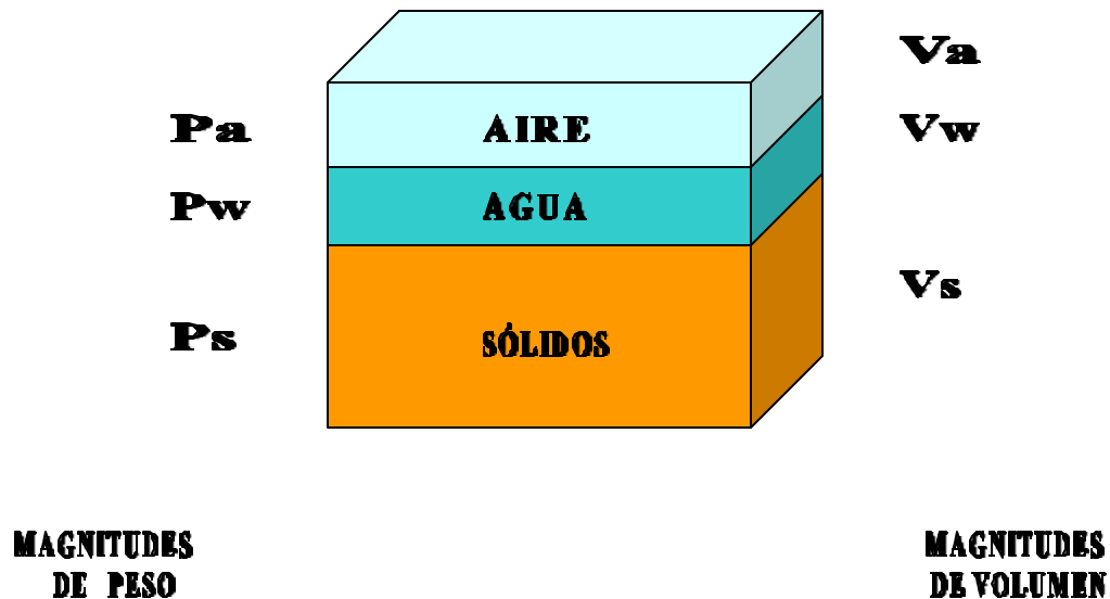
FIGURA 6.4. Componentes gravimétricos y volumétricos básicos del suelo.
