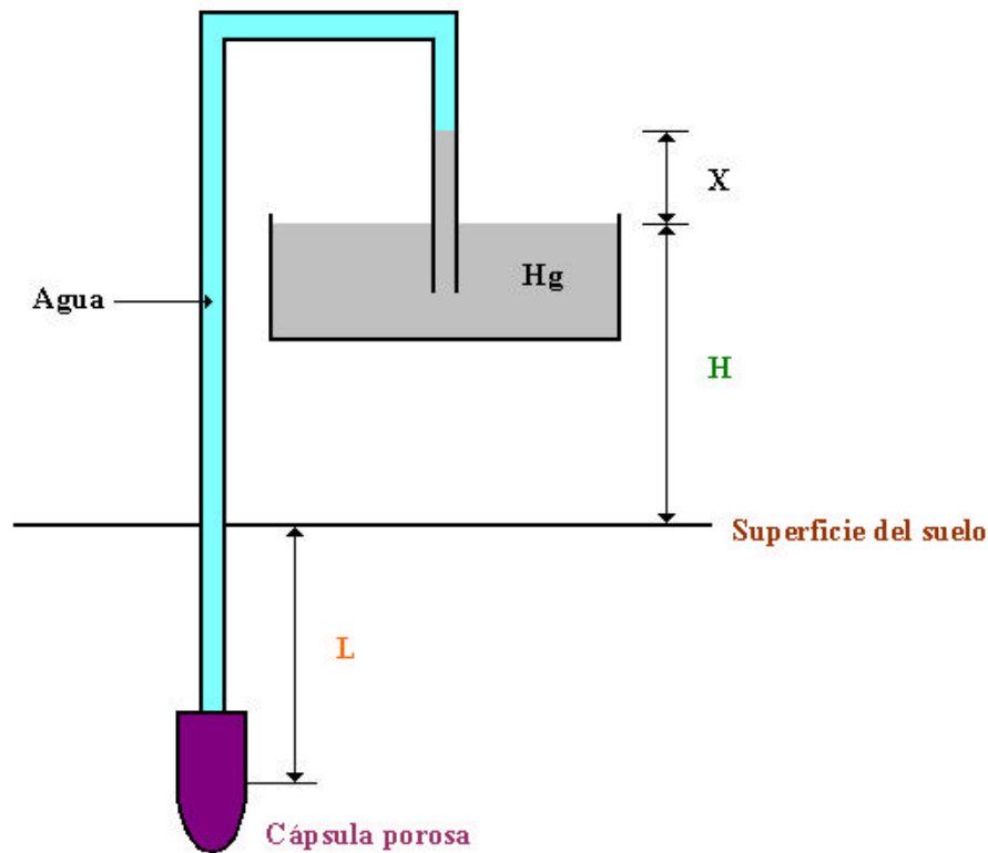
FIGURA 9.6. Representación esquemática de un tensiómetro de mercurio.
