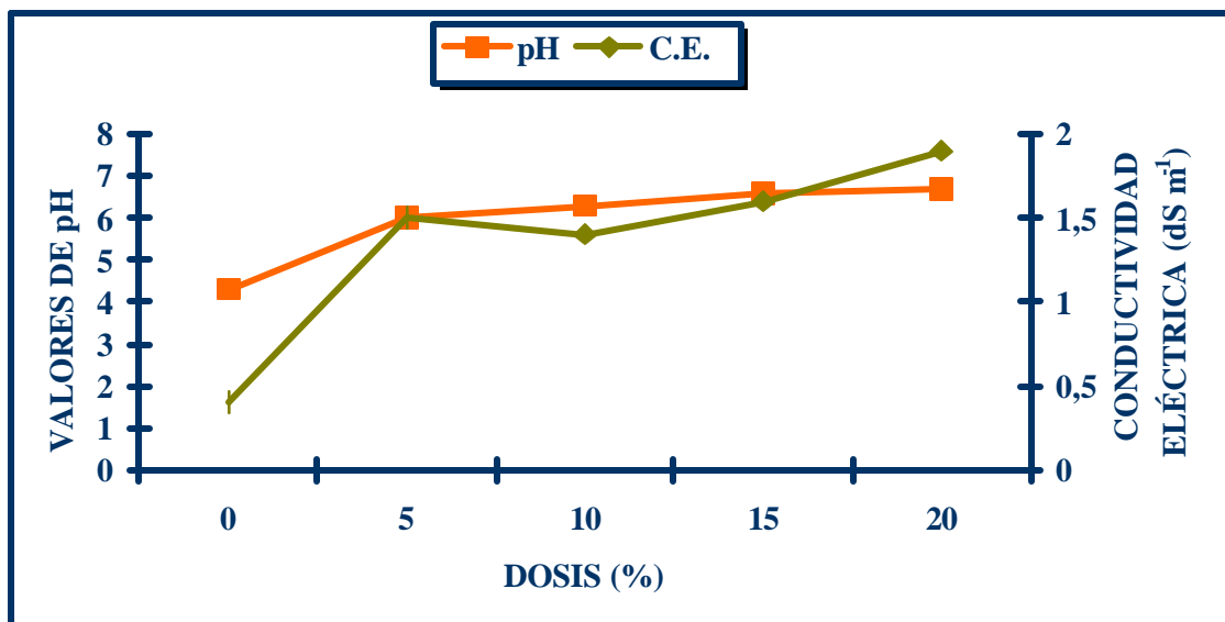
FIGURA 17.4. Efecto de la adición de lodos de plantas de tratamiento de aguas residuales urbanas del municipio de El Retiro, oriente antioqueño, sobre el pH y la salinidad de un Ultisol muy ácido y muy pobre del valle de Aburrá (Antioquia). (Con base en resultados de Gutiérrez et al, 1998).
