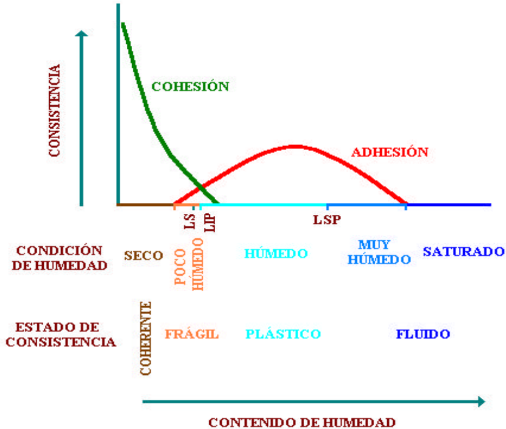
FIGURA 10.1. Efecto de la humedad en la consistencia del suelo (comp lementado de Mejía, 1980).
