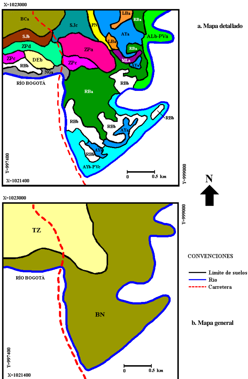
FIGURA 21.2. Fragmentos de mapas de estudios de suelos, con diferente detalle, de un sector de la Sabana de Bogotá. a. De un estudio detallado (Tomado de IGAC, 1977). b. De un estudio general (Tomado de Carrera et al, 1968).
