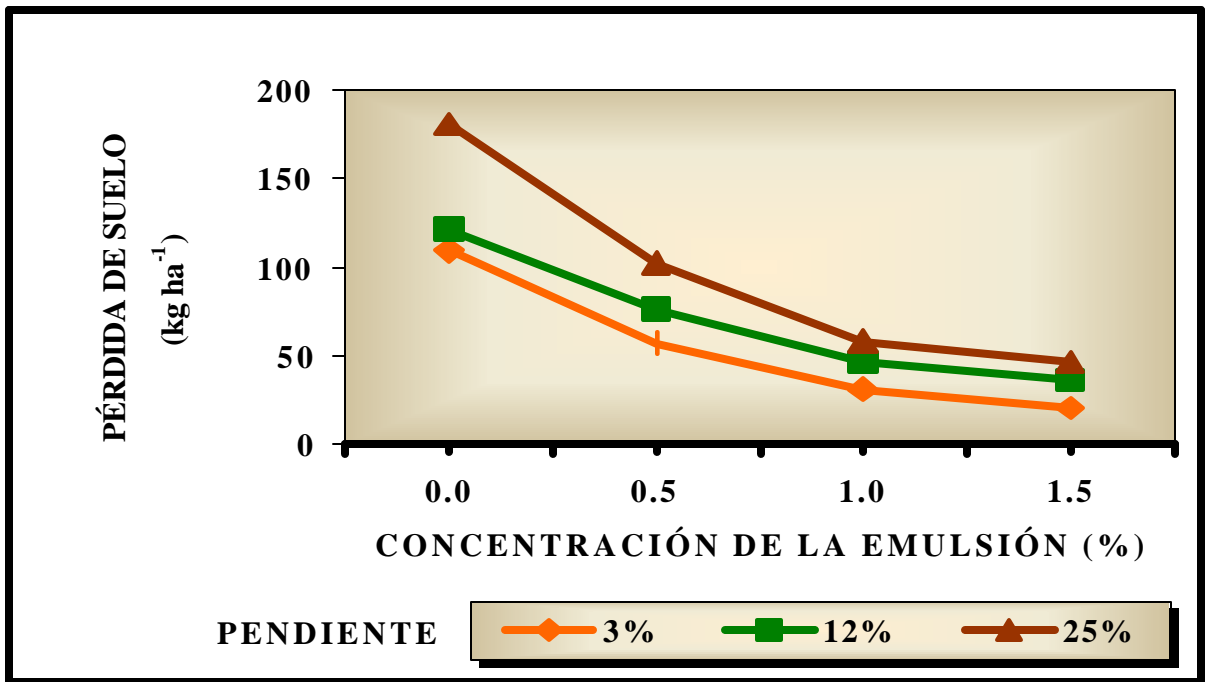
FIGURA 11.11. Efecto de la aplicación de emulsión asfáltica en la pérdida de suelo por escorrentía superficial en un Dystric Haplustand medial isomésico de la Sabana de Bogotá, sometido a una lluvia artificial de 68 mm h -1 de intensidad, durante 30 minutos. (Con base en resultados de González et al, 1993).
