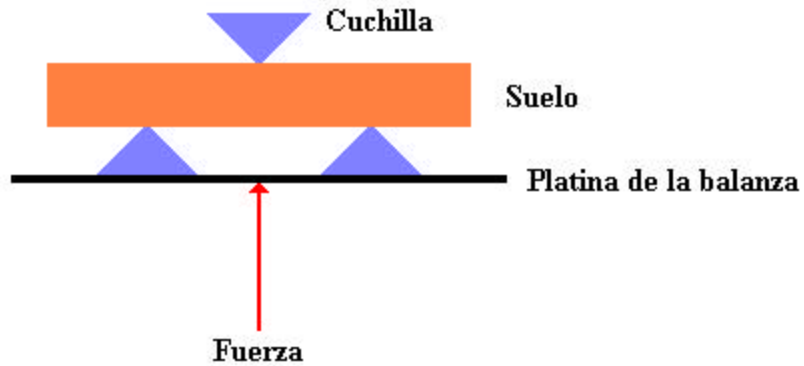
FIGURA 10.3. Representación de la disposición de los materiales utilizados para determinar el módulo de ruptura del suelo por el método de Richards.
