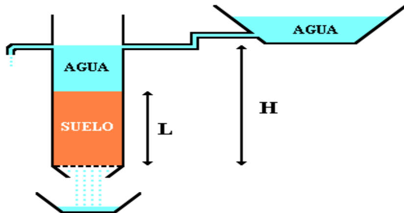
FIGURA 9.16. Representación esquemática de un permeámetro de cabeza constante.
