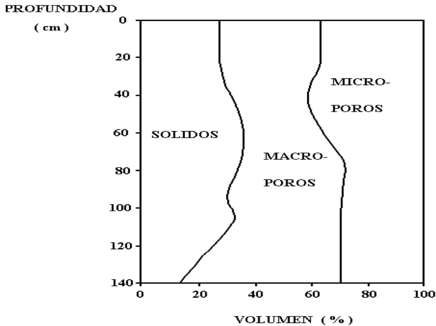
FIGURA 8.7. Variación de la distribución de la porosidad en un Typic Dystrandepht medial isomésico, con la profundidad del suelo. (Con base en datos de IGAC, 1977).
