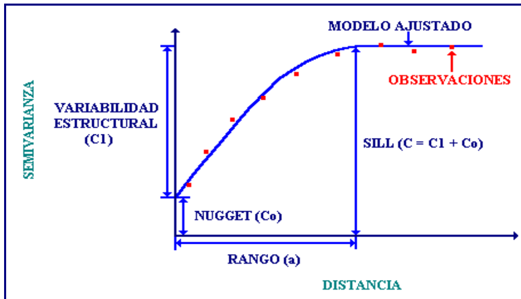
FIGURA 23.2. Ejemplo hipotético de un semi variograma con sus componentes.
