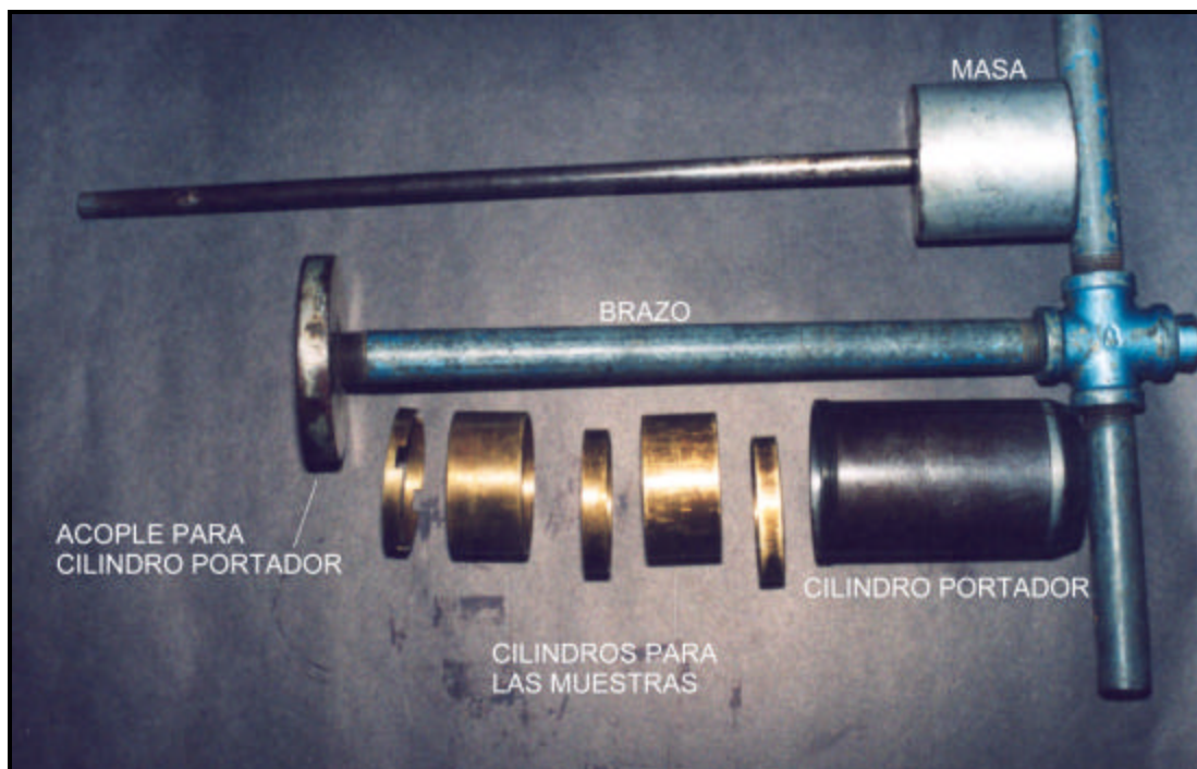
FIGURA 8.4. Barreno para tomar muestras de suelo sin disturbar.
