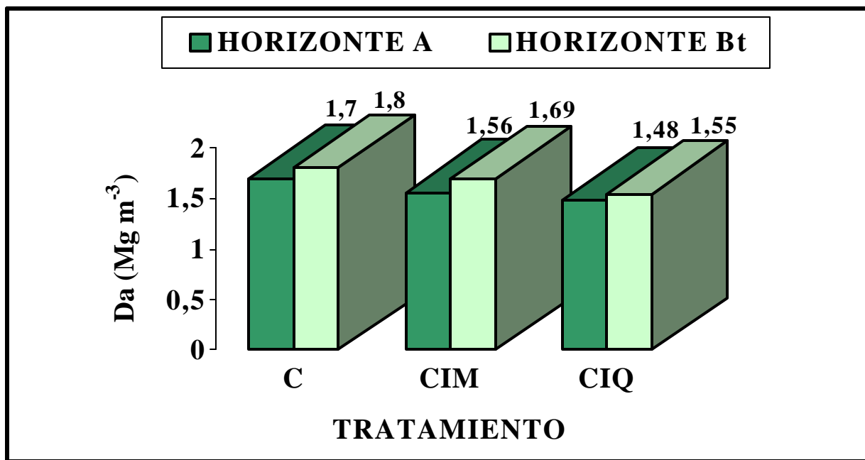
FIGURA 11.2. Efecto de diferentes métodos de labranza sobre la densidad aparente de los horizontes A (0-18 cm) y Bt (18-40 cm) de un Arenic Haplustalf de El Espinal (Tolima). C: Labranza convencional; CIM: Labranza profunda con cincel, incorporando cascarilla de arroz; CIQ: Labranza reducida profunda con cincel y control de malezas con herbicida. (Con base en resultados de Castro y Amézquita, 1991).
