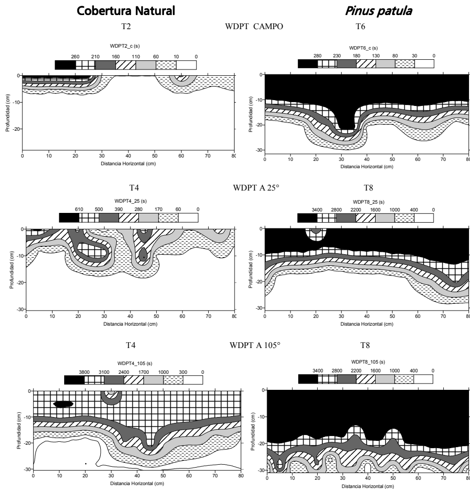
Figura 4. Variabilidad espacial del WDPT con la profundidad, para transectos representativos muestreados en las diferentes coberturas en andisoles de Antioquia, Colombia (transecto 2: con dirección E-O y en época seca, transecto 6: con dirección E-O y en época seca, transecto 4: con dirección E-O y en época húmeda y transecto 8: con dirección E-O y en época húmeda), en condiciones de campo y con muestras secadas a 25 y 105°C. (Adaptada de Vanegas, 2003).
