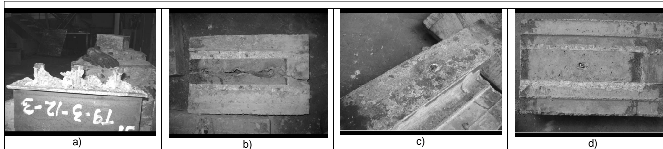
Figura 4. a) Estado final de los conectores en la falla del concreto. b) Estado final de la placa de concreto. c) Estado final del perfil metálico en la falla de la soldadura. d) Tornillo embebido en la placa de concreto ante la falla de la soldadura. (Tomado de Hurtado, 2005).
