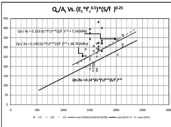
(DSVE – Datos sin valores extremos, DCVE – Datos con valores extremos). Figura 8. Regresión, planteamiento general de diseño.
