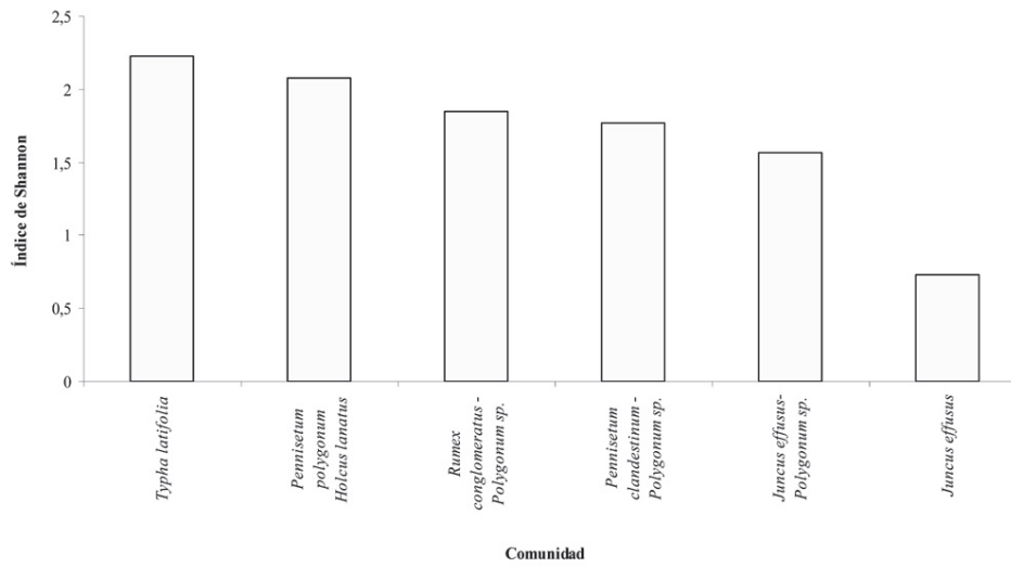
Figura 5. Índices de diversidad de Shannon.
