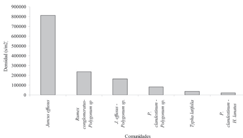
Figura 2. Densidad total de semillas para los diferentes parches de vegetación del humedal Jaboque.
