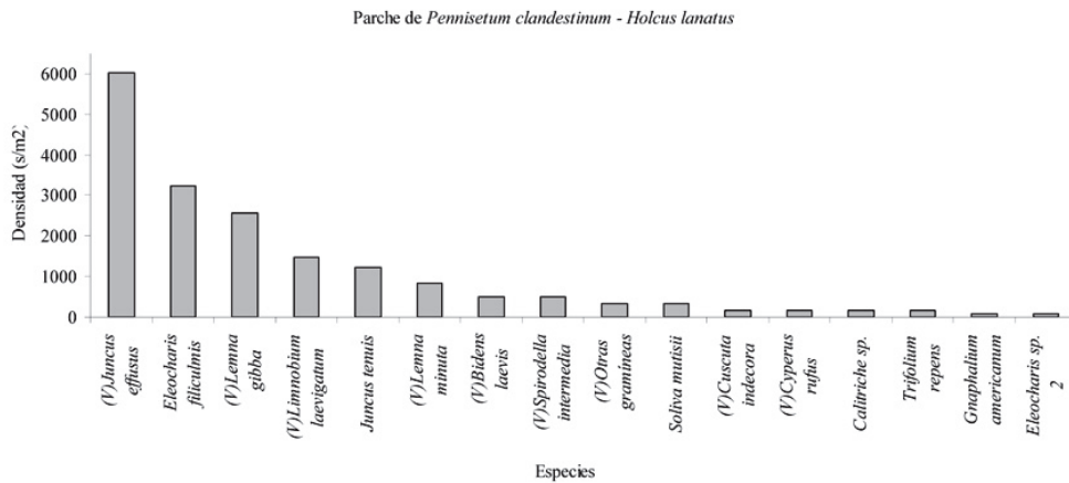
Continuación Figura 3. Densidad de semillas por especie para los parches de vegetación, (V) especies presentes en la vegetación. Patrones de abundancia.
