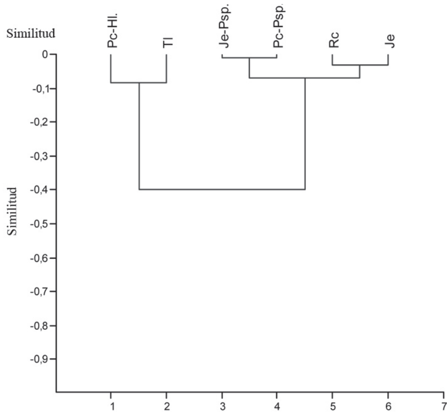
Figura 6. Similitud entre el Banco de semillas y la vegetación del humedal Jaboque (Índice de Sørensen).
