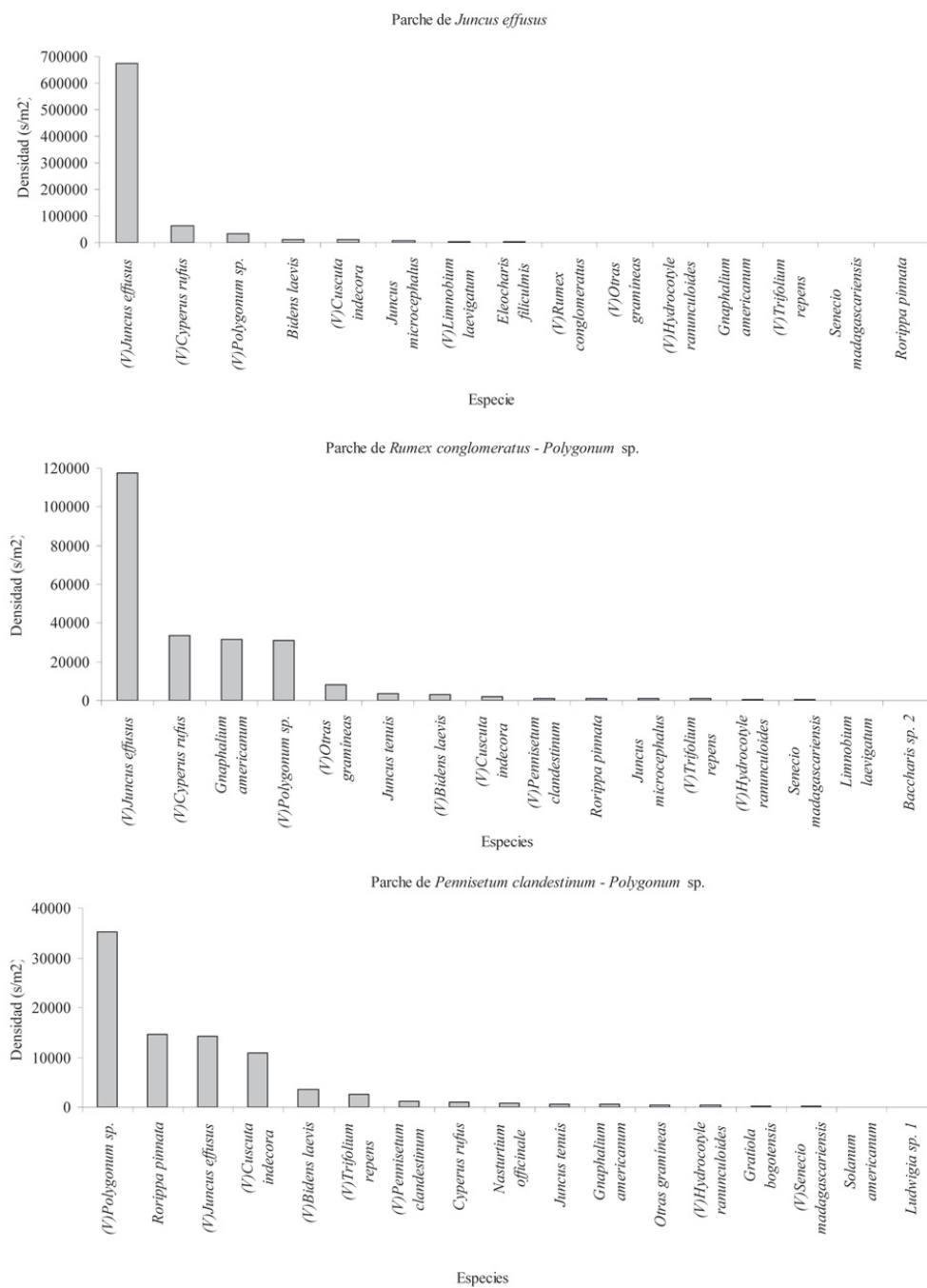
Figura 3. Densidad de semillas por especie para los parches de vegetación, (V) especies presentes en la vegetación. Patrones de abundancia.
