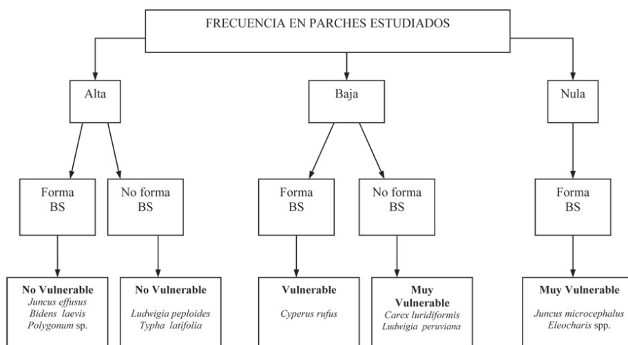
Figura 7. Vulnerabilidad de las especies propias del humedal Jaboque. BS: Banco de Semillas.
