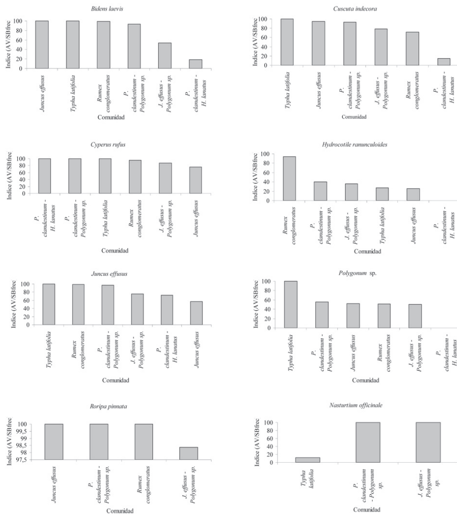
Figura 4. Persistencia de las especies más comunes del banco de semillas en el Humedal Jaboque.
