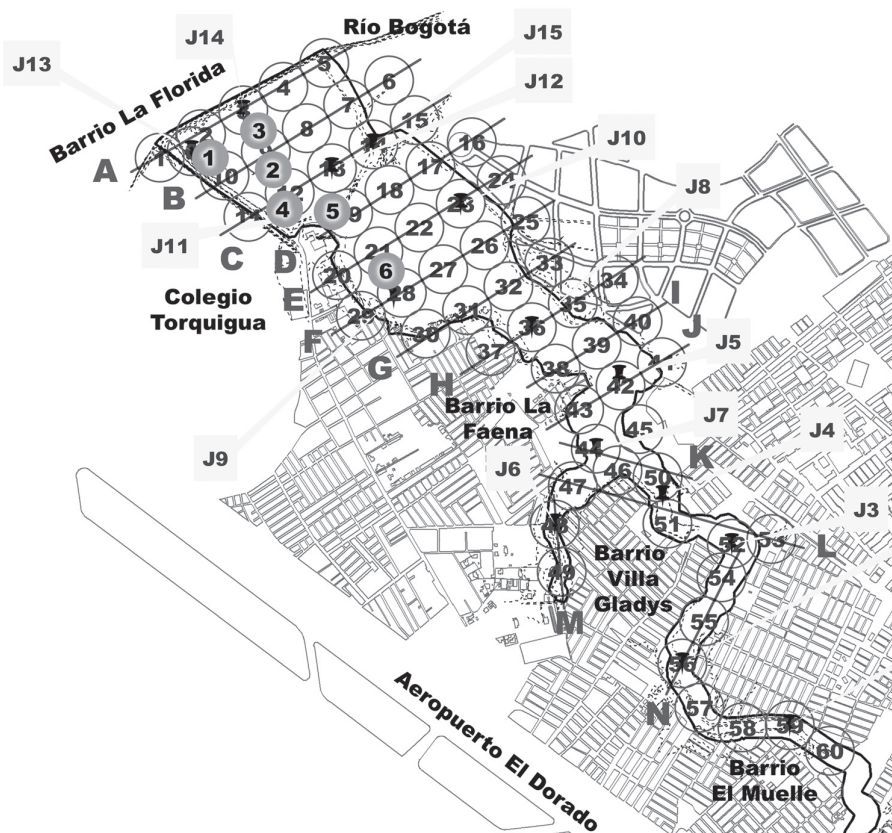
Figura 1. Mapa del humedal Jaboque (diseño H. Arellano). Puntos de muestreo del banco de semillas en las comunidades de: 1. Juncus effusus - Polygonum sp., 2. Rumex conglomeratus - Polygonum sp. 3. Typha latifolia . 4. Pennisetum clandestinum - Holcus lanatus . 5. Juncus effusus . 6. Pennisetum clandestinum - Polygonum sp.
