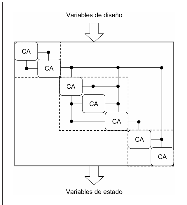
Figura 4. Distribución diagonal de subsistemas con una interconexión matricial ordenada. En este esquema híbrido los clusters (representados por líneas punteadas) están organizados en un esquema jerárquico; los subsistemas en cada cluster tienen una organización no jerárquica
