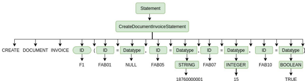
Figura 3-14.: AST Ejemplo 3. Creación de un documento tipo factura. Fuente: Propia.
