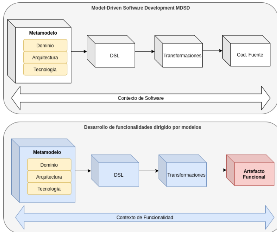
Figura 2-5.: Desarrollo de funcionalidades dirigido por modelos. Fuente: Imagen propia
