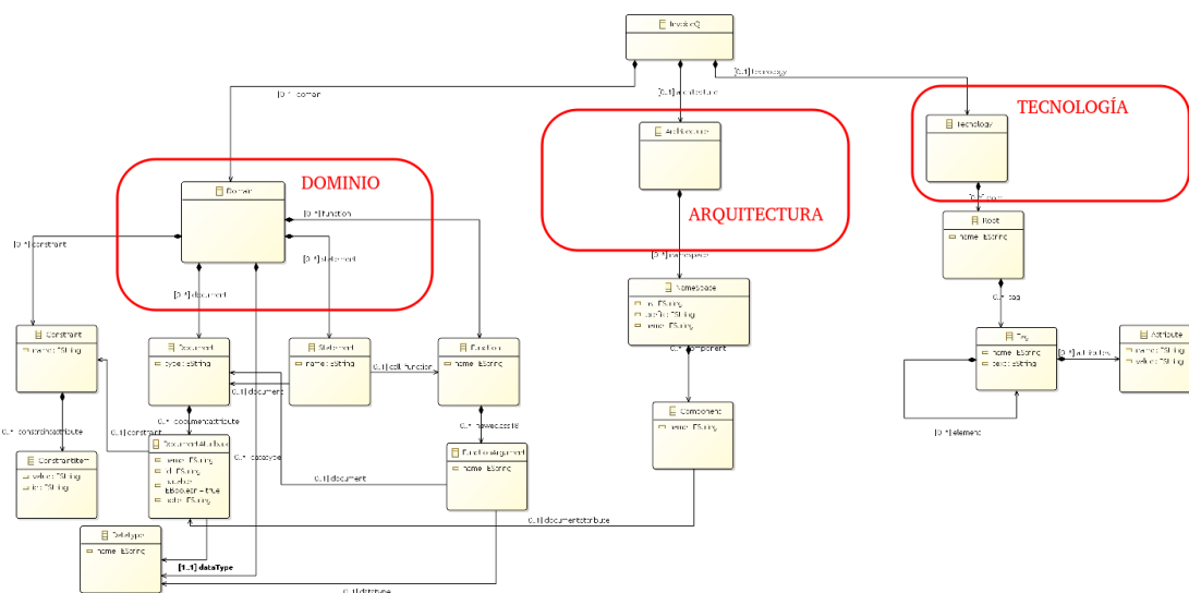
Figura 3-4.: Ramas del metamodelo. Fuente: Propia.
