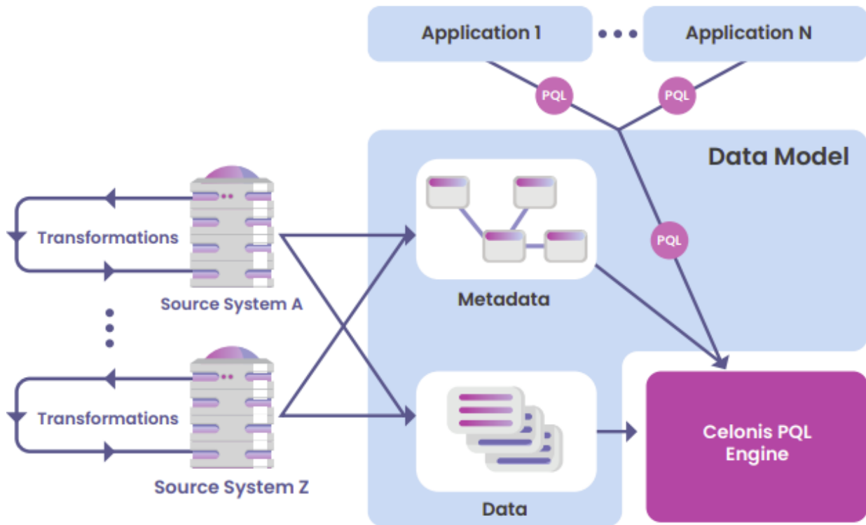
Figura 2-9.: Arquitectura de Celonis PQL. Fuente: Vogelgesang(2019)[21]
