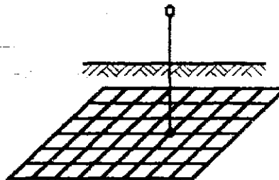
d. toma de tierra de red en malla
