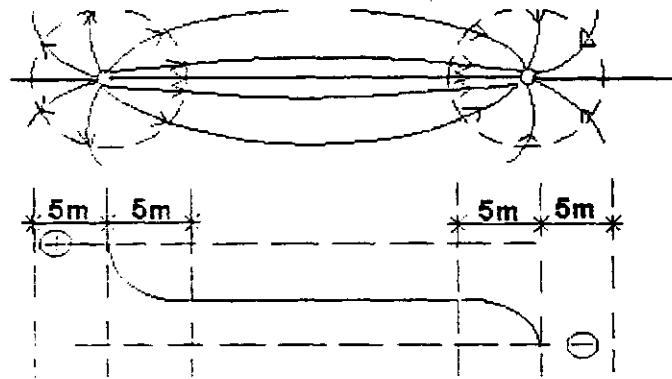
b. Gradientes de tensión entre dos electrodos
