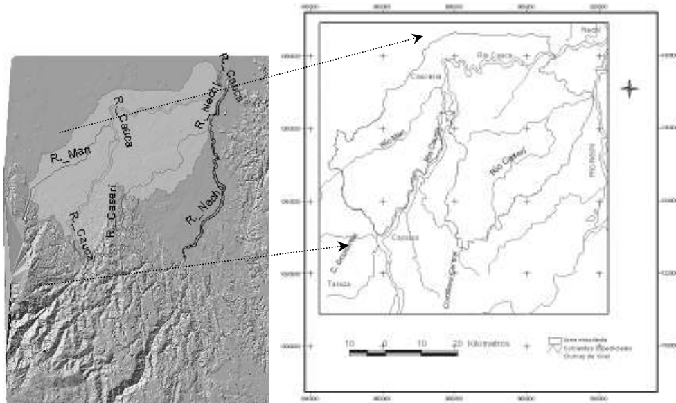
Figura 1. Localización del área de estudio Figure 1. Localization
