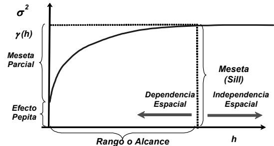
Figura 4. Principales elementos del Variograma. (Mejía, 2006)
