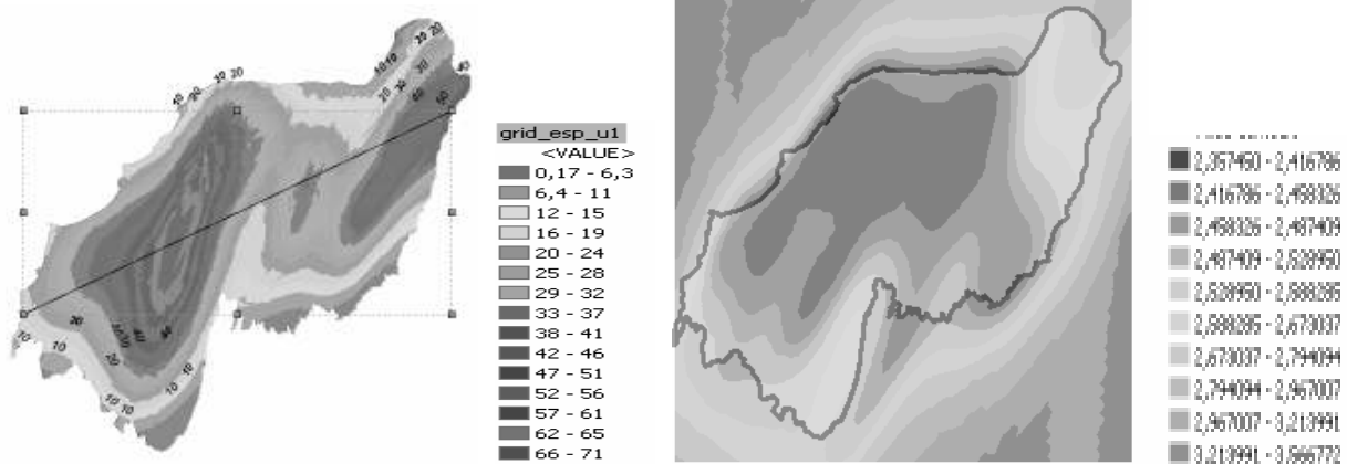
Figura 5. Superficie raster de predicción de los espesores de la Unidad acuífera U 123 obtenida mediante Modelo Gaussiano y Mapa de error estimado de la predicción.
