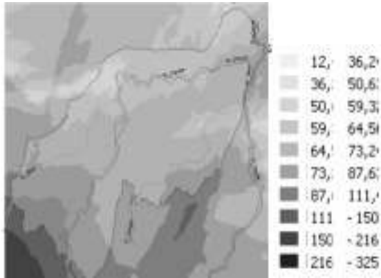
Figura 10. Superficie piezométrica de la Unidad acuífera U_{123} . Kriging ordinario y Modelo Gaussiano. Figure 10. Freatic surface to U_{123}
