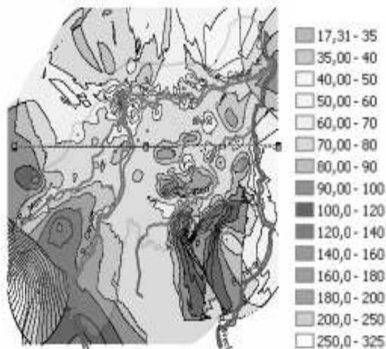
Figura 11. Superficie piezométrica y Líneas equipotenciales de la Unidad U_{123} . Figure 11. Freatic surface and equipotential lines to U_{123}
