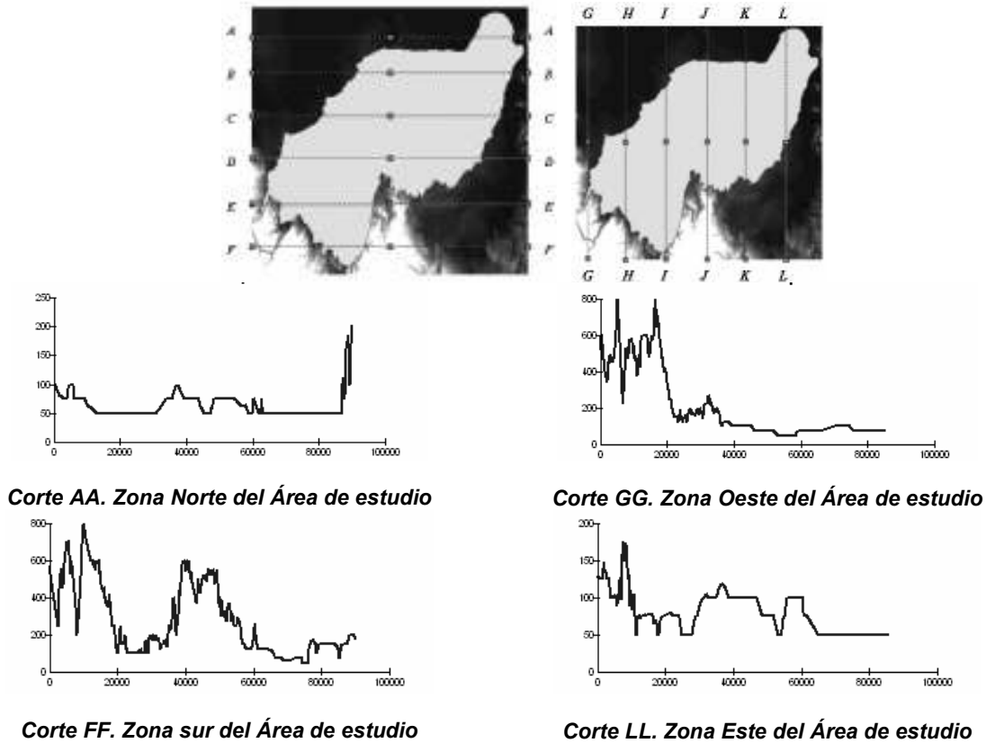
Figura 2. Comportamiento hipsométrico del área de estudio en las direcciones Este oeste y Norte Sur. Figure 2. Hypsometric and cross sections
