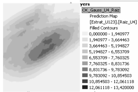
Figura 8. Superficie resultante a partir de Kriging para la Unidad acuífera U 4 .
