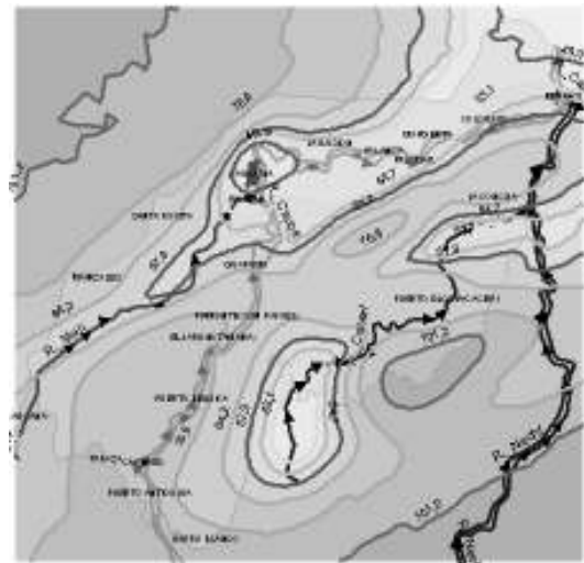
Figura 12. Superficie piezométrica final de la Unidad acuífera U_{123} . Figure 12. Final freatic surface to U_{123}
