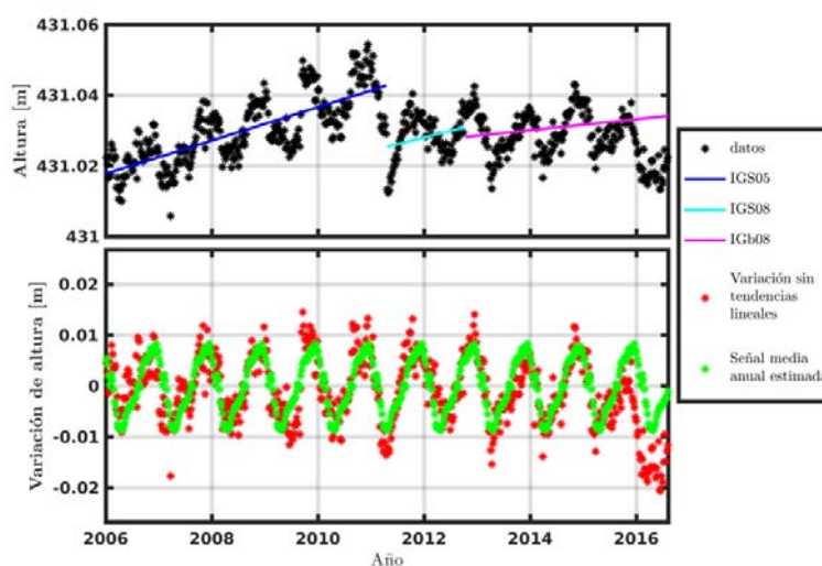
Figura 13. Preprocesamiento de la componente vertical de la estación PPT. Figure 13. Preprocessing of PPT vertical component.
