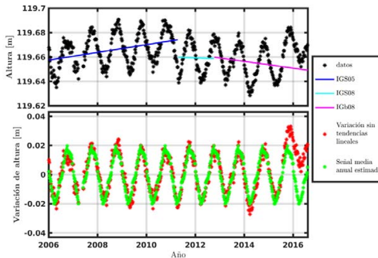
Figura 12. Preprocesamiento de la componente vertical de la estación POVE.
