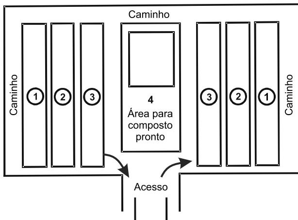
Figura 4. Disposição e formação da pilha.
