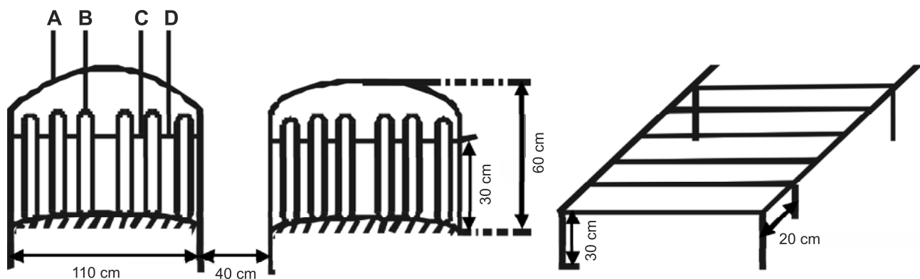
Figura 6. Tiras de bambu (A); tubos (B); estrutura de suporte (C); superfície convexa (D).
