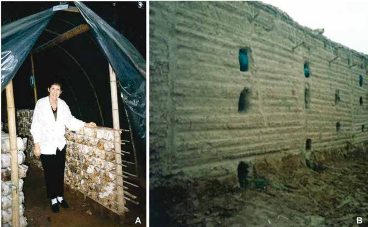
Figura 9. Cogumelos cultivados com a técnica JunCao em barracas de lona, em Fujian, na China (A); galpão de argila em Yanchuan, na China (B).
