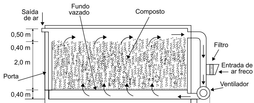
Figura 10. Câmara de pasteurização.
