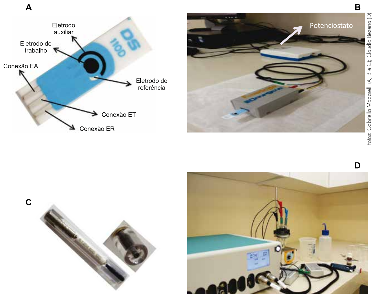
Figura 4. Eletrodo impresso (A) e sistema portátil - potenciostato, conexões e eletrodo impresso (B); eletrodo de trabalho convencional ( \phi = 2,0 mm) (C) e potenciostato convencional conectado à célula eletroquímica (D). Potenciostatos são geralmente usados para análises voltamétricas.
