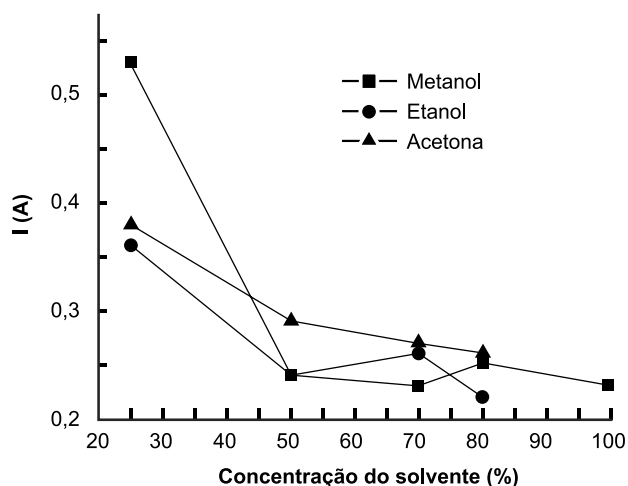
Figura 6. Correntes máximas de oxidação I (A) na faixa de potencial de 0,8 V obtidas da análise da amostra liofilizada de cogumelo da espécie Pleurotus ostreatus por método voltamétrico, submetida a extração pelos solventes etanol, metanol e acetona, em diferentes concentrações (%). Fonte: Cavalcante (2013) e Magarelli (2014).
