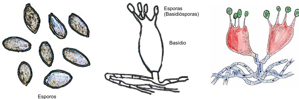
Figura 2. Desenhos esquemáticos de esporos e basídios de cogumelo.
