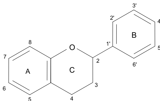
Figura 2. Estrutura química geral dos flavonoides.
