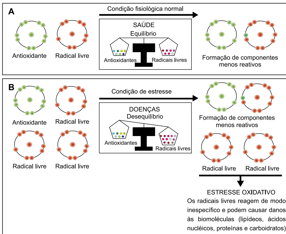
Figura 3. Esquema simplificado: (A) condição fisiológica normal; (B) condição de estresse (estresse oxidativo).
