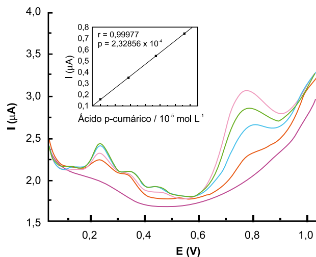
Figura 7. Voltamogramas de pulso diferencial de 750 µL do extrato de cogumelo Ganoderma lucidum (vermelho) em tampão fosfato pH 4 (preto), com três adições padrões de ácido p-cumárico (em azul) nas concentrações de 3,4 \times 10^{-5}M ; 7,3 \times 10^{-5}M e 14,5 \times 10^{-5}M . Parâmetros eletroquímicos: velocidade de varredura de 50 mV/s; amplitude de pulso de 50 mV. Eletrodo de trabalho: carbono vítreo. Eletrodo de referência: prata/cloreto de prata (Ag/AgCl). Eletrodo auxiliar: platina (Pt). Inserção: curva de adição padrão com o coeficiente de correlação.
