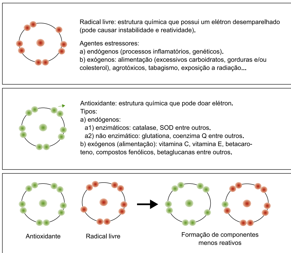
Figura 2. Esquema simplificado (diferença entre radical livre e antioxidante).
