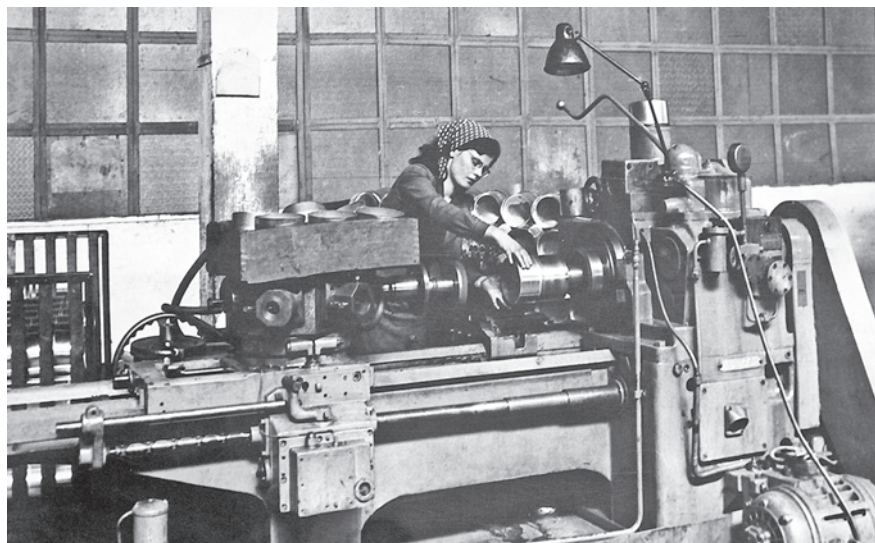
Munkásnő az esztergapadnál
