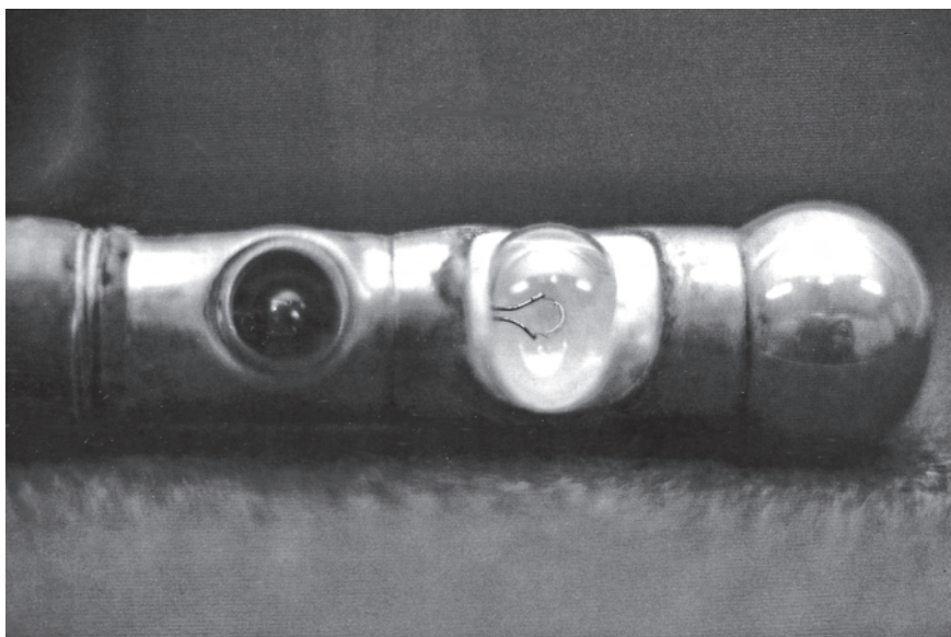
Az elsőként használt Wolf-Schindler-féle fűlmerev gasztroszkóp optikája
