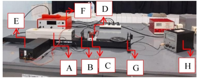
Gambar 1. Set up alat pengukuran sudut rotasi Faraday
