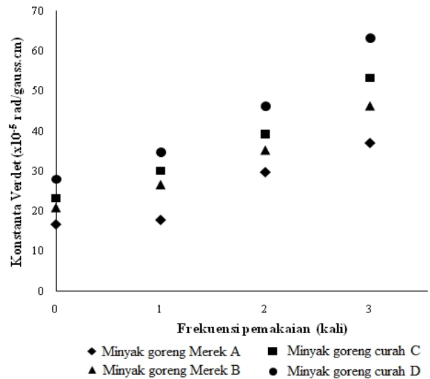
Gambar 2. Grafik hubungan frekuensi pemakaian minyak goreng dengan konstanta Verdet
