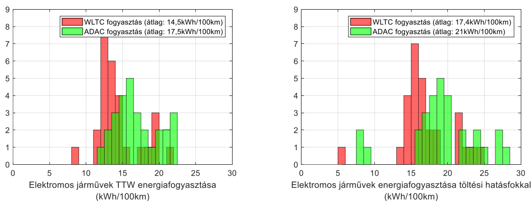
2. ábra. Akkumulátoros elektromos személygépjárművek energiafogyasztásainak WLTC menetciklus és ADAC mérések [3] szerinti összehasonlítása
