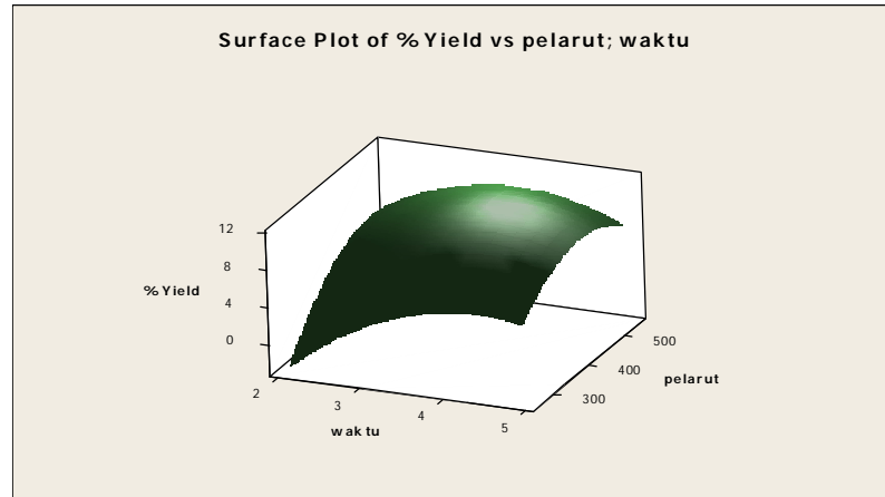
Gambar 1. Surface Plot Pengaruh Waktu dan Pelarut terhadap Yield
