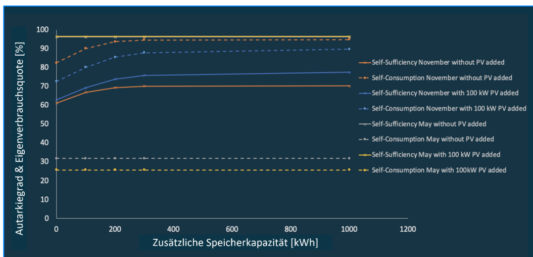
Abbildung 4: Eigenverbrauch und Autarkie mit zusätzlicher Speicherkapazität
