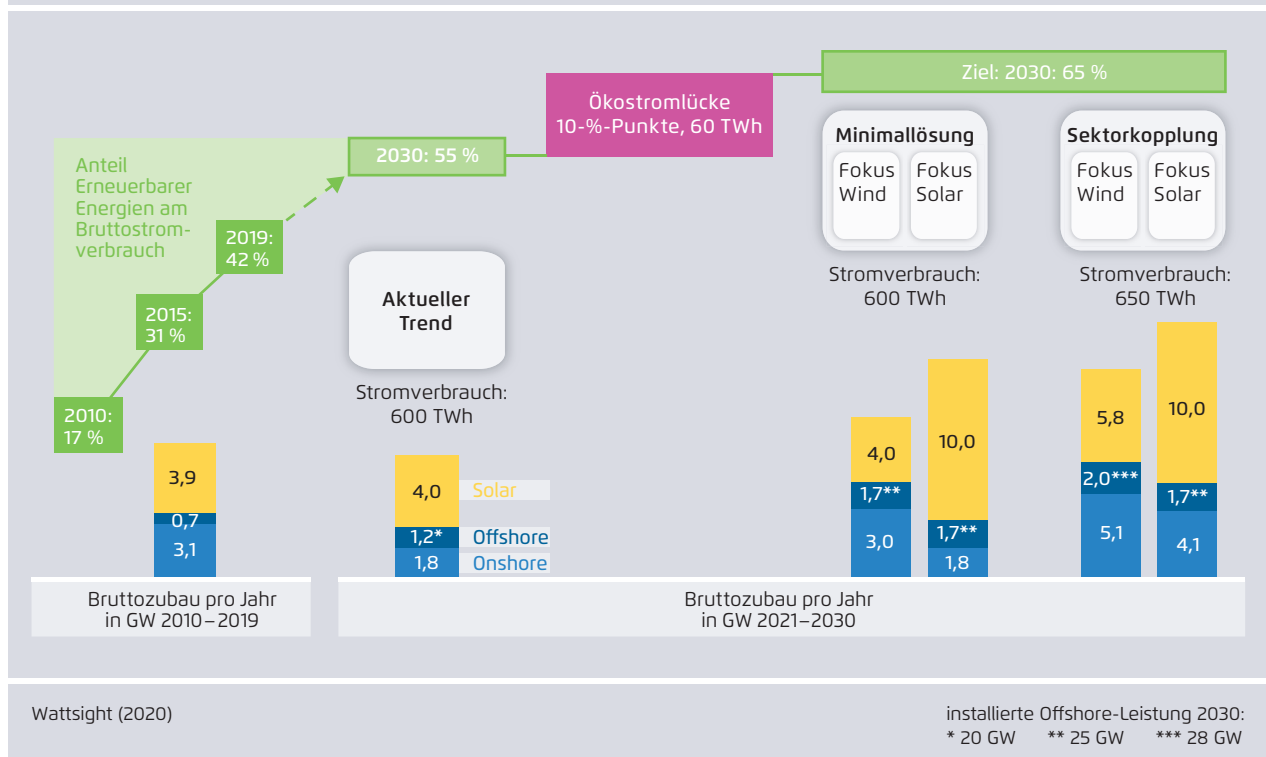
Anteil Erneuerbarer Energien 2010 bis 2030 sowie durchschnittlicher Bruttozubau von Windenergieleistung an Land und auf See sowie von Photovoltaikleistung im Zeitraum 2010 bis 2019 und von 2021 bis 2030
