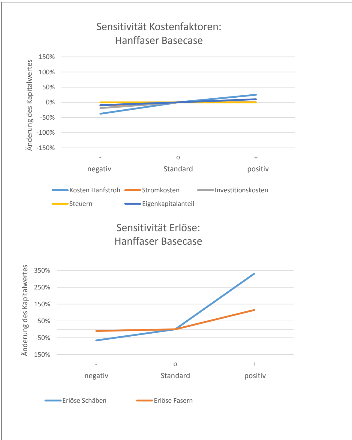
Abb. 9.4: Ergebnisse der Sensitivitätsanalysen – Hanffaseraufschluss Base Case
