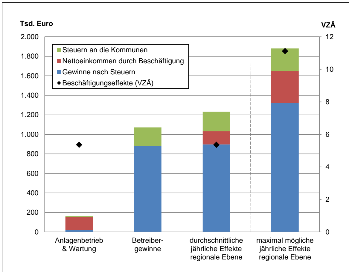
Abb. 5.4: Regionale Wertschöpfung und Beschäftigung der Biogaserzeugung mit Gärrestaufbereitung in einer fiktiven Beispielregion, jährliche Effekte (Basisjahr 2016)
