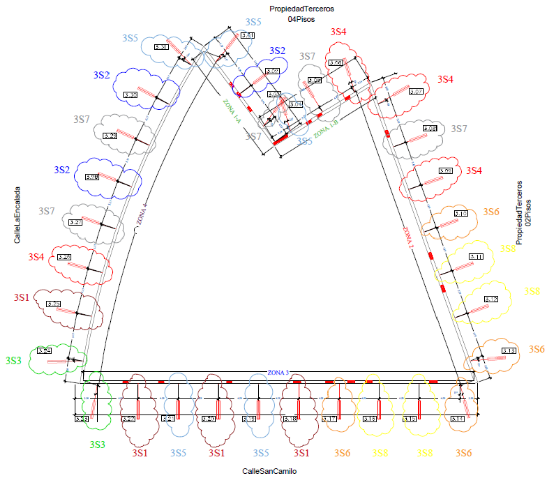
Figura 8: Sectorización Tercer anillo.
