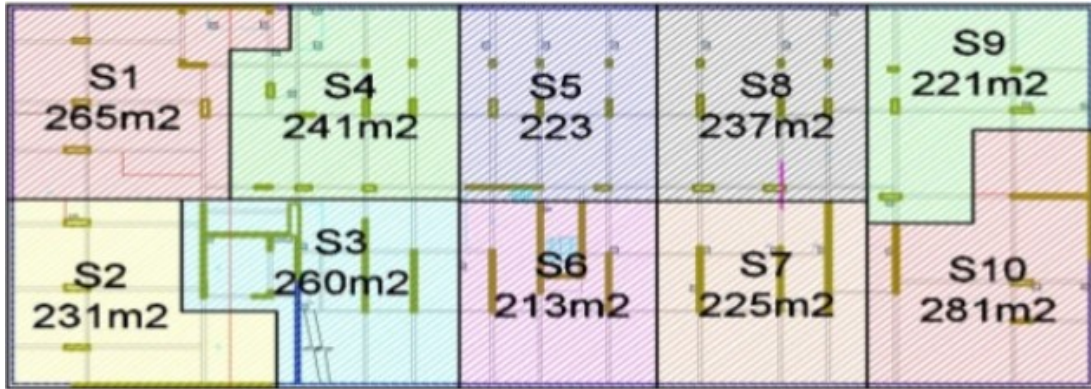
Figura 2: Sectorización de sótanos de un edificio multifamiliar de 17 niveles con 4 sótanos [6].
