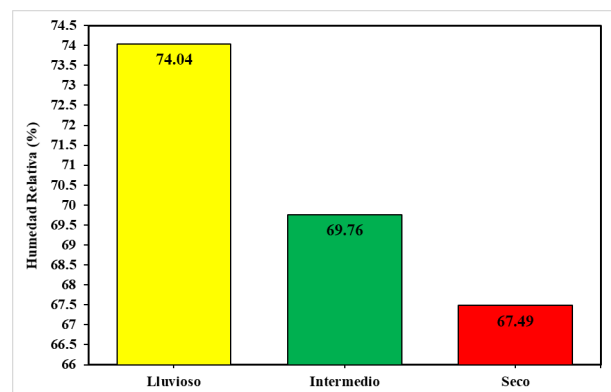
Figura 9: Estadíos de la Humedad Relativa en la microcuenca Apacheta.
