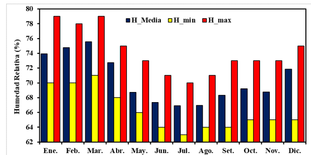
Figura 8: Distribución estacional de la Humedad Relativa Media mensual, mínima y máxima, microcuenca Apacheta.
