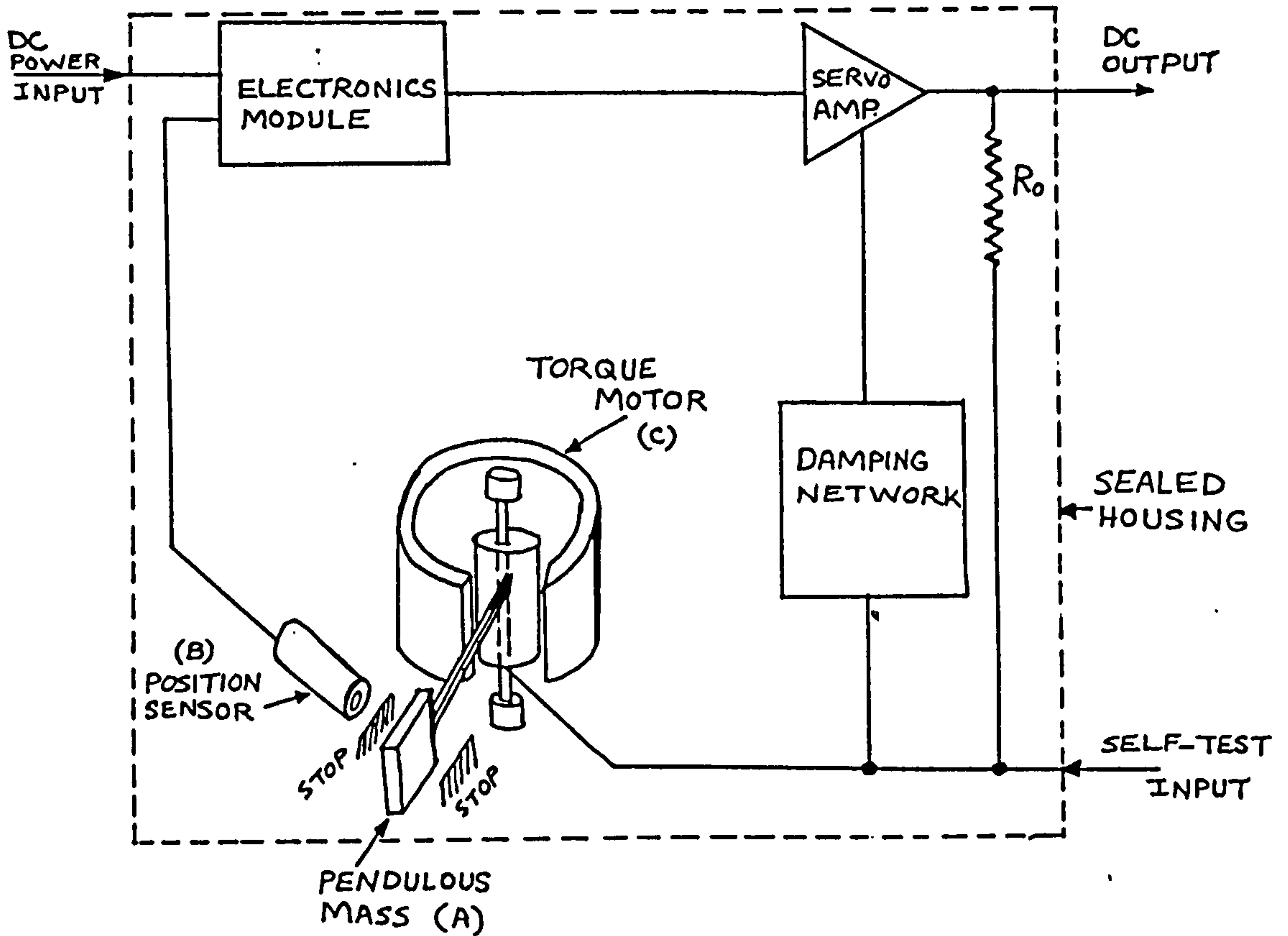
FIG. 5.1 LINEAR SERVO ACCELEROMETER
