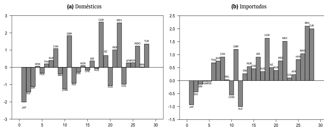
Figura 5. Betas incondicionais.
