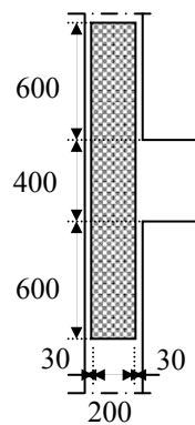
Σχήμα 4. Τοποθέτηση των διαγώνιων υφασμάτων
