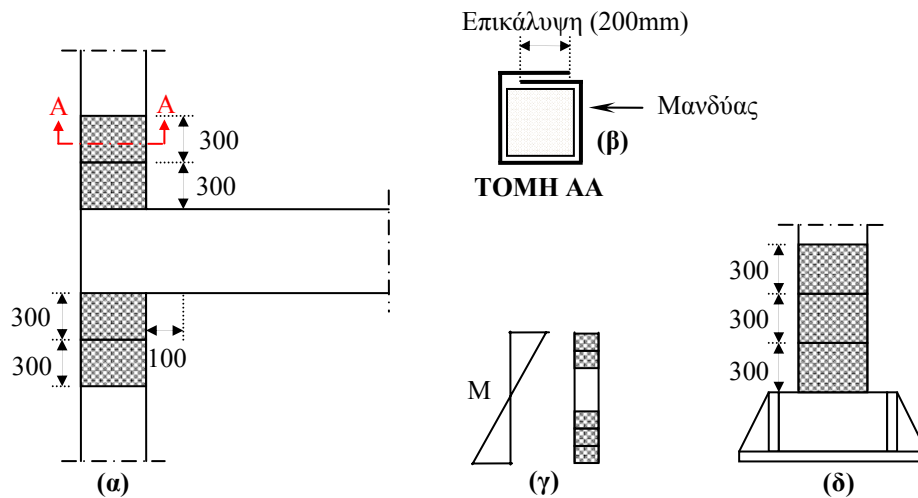
Σχήμα 7. Περίσφιγξη των υποστρωμάτων (Chaudat et al., 2005)
