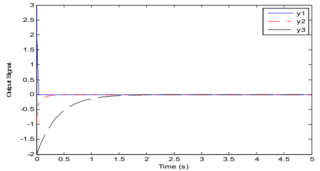
图1:单输入静态反馈控制的Lorenz混沌系统响应曲线
