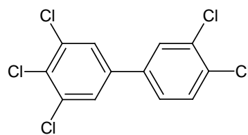
3,3',4,4',5-pentachlorobiphenyl (PCB126)
