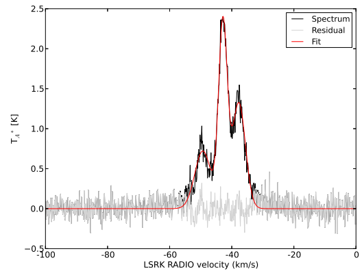
(d) HCN
