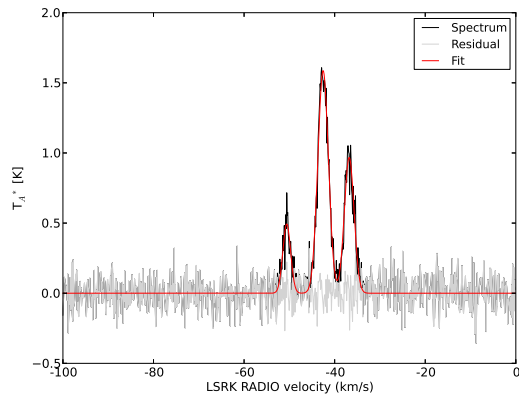
(a) \text{N}_2\text{H}^+
