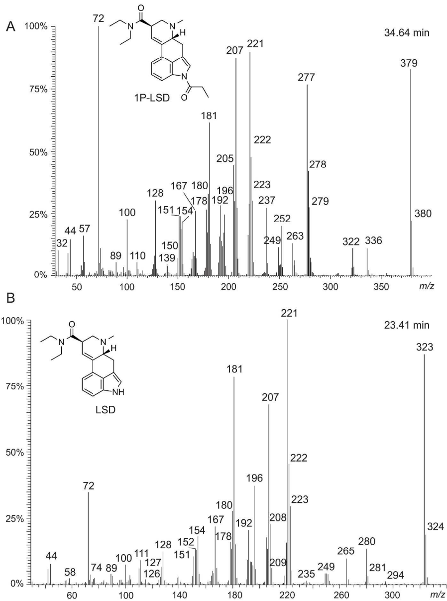
Figure 2. Electron ionization quadrupole mass spectra. A: 1P-LSD. B: LSD 266x355mm (300 x 300 DPI)
