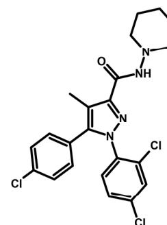
Rimonabant
