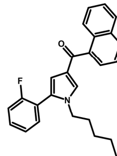
JWH-307
