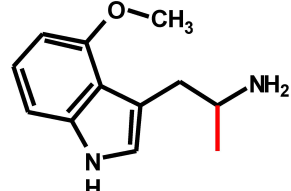
4-MeO-AMT
