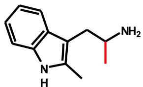
2-Me-AMT
