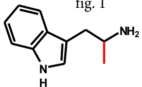
AMT
