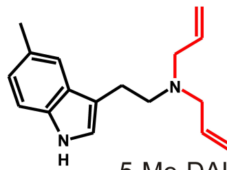
5-Me-DALT
