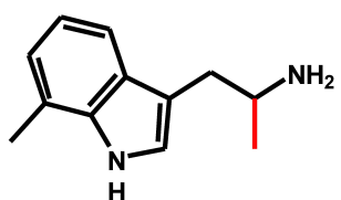
7-Me-AMT
