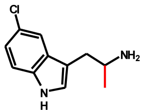
5-Cl-AMT
