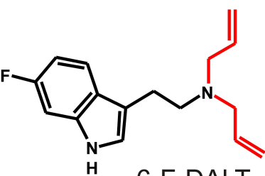
6-F-DALT
