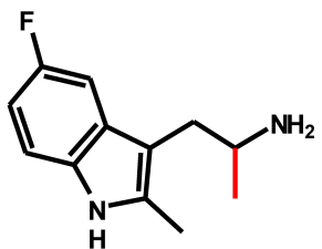
5-F-2-Me-AMT
