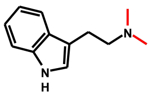
DMT
