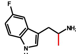
5-F-AMT
