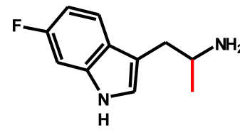
6-F-AMT
