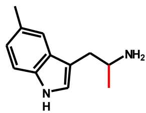
5-Me-AMT
