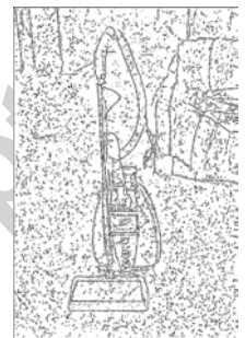
(j) Kovesi
