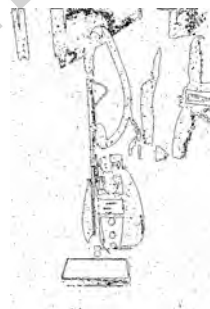
(n) TCA 112
